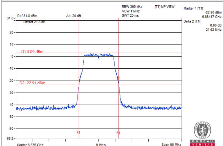
802.11a / Chain 0 : CH 185
