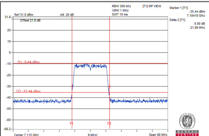
802.11ax (HE20) / Chain 0 : CH 233
