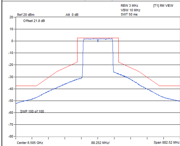
802.11ax (HE160) / Chain 1 : CH 111
