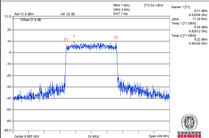
802.11ax (HE80) / Chain 1 : CH 183
