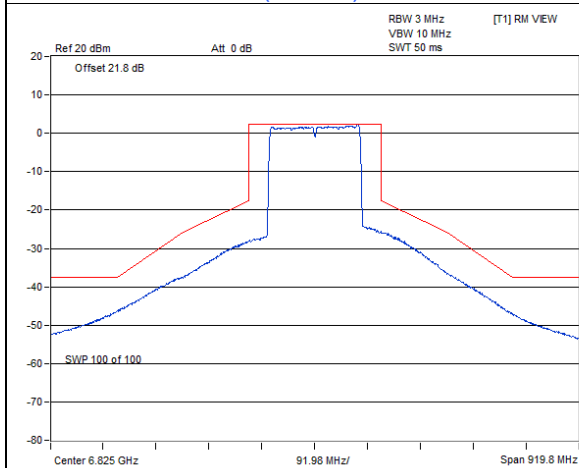
802.11ax (HE160) / Chain 1 : CH 175
