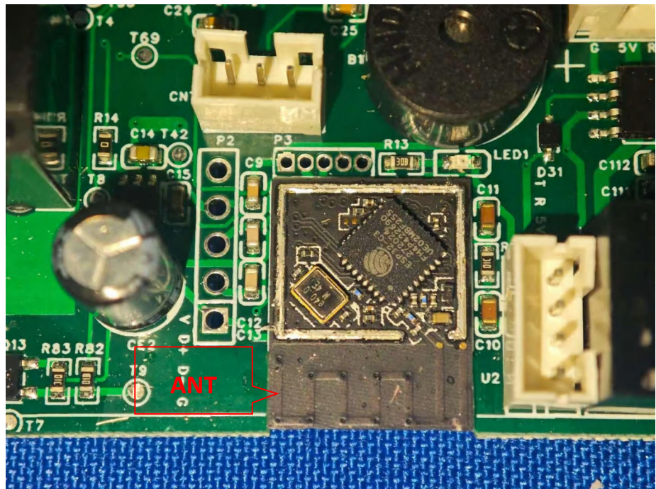
EUT Photo 17
