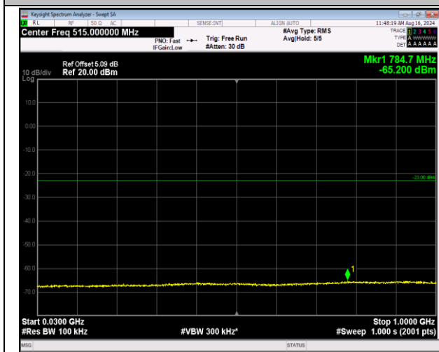
66-66-5MHz-20MHz-16QAM-16QAM-132330-132447-1R B#0-1RB#99-30~1000MHz-PASS
