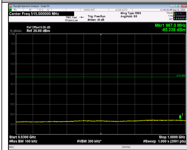
66-66-5MHz-20MHz-QPSK-QPSK-132330-132447-1RB# 24-0RB#0-30-1000MHz-PASS
