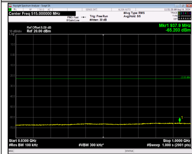
66-66-5MHz-20MHz-QPSK-QPSK-132455-132572-1RB# 24-0RB#0-30~1000MHz-PASS
