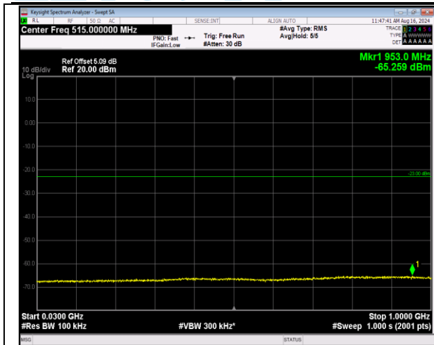
66-66-5MHz-20MHz-QPSK-QPSK-132330-132447-1RB# 0-1RB#99-30-1000MHz-PASS
