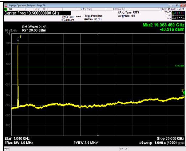
66-66-5MHz-20MHz-QPSK-QPSK-132005-132122-1RB#0- 1RB#99-1000~20000MHz-PASS
