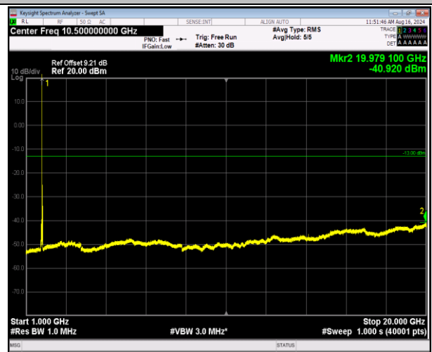
66-66-5MHz-20MHz-QPSK-QPSK-132455-132572-1RB#24 -0RB#0-1000~20000MHz-PASS
