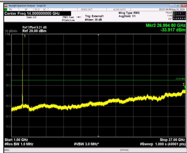
41-41-20MHz-20MHz-QPSK-QPSK-41292-41490-1RB#99- 0RB#0-1000~27000MHz-PASS
