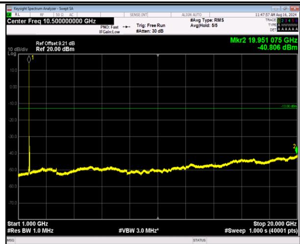
66-66-5MHz-20MHz-QPSK-QPSK-132330-132447-1RB#0- 1RB#99-1000-20000MHz-PASS
