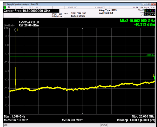
66-66-5MHz-20MHz-QPSK-QPSK-132455-132572-25RB#0 -100RB#0-1000~20000MHz-PASS
