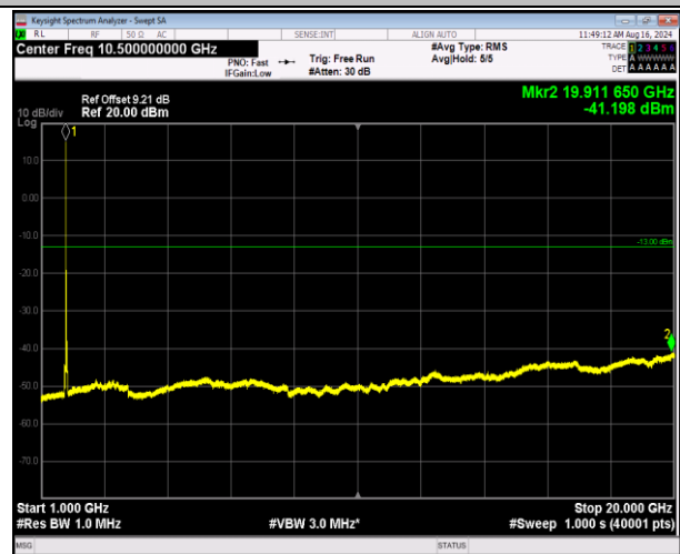
66-66-5MHz-20MHz-QPSK-QPSK-132330-132447-25RB#0 -100RB#0-1000-20000MHz-PASS
