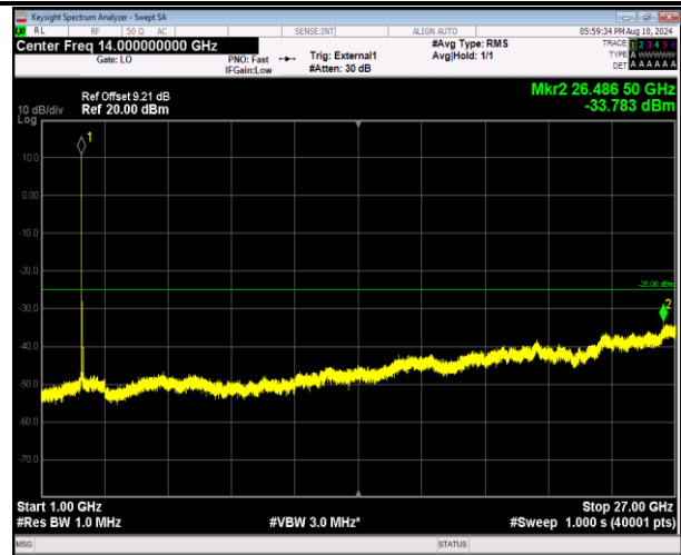
41-41-20MHz-20MHz-QPSK-QPSK-41292-41490-1RB#0-1 RB#99-1000~27000MHz-PASS
