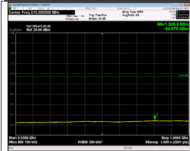
66-66-5MHz-20MHz-QPSK-QPSK-132455-132572-1RB# 0-1RB#99-30~1000MHz-PASS
