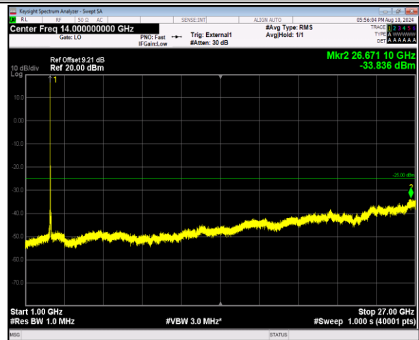
41-41-20MHz-20MHz-QPSK-QPSK-41292-41490-1RB#0-0 RB#0-1000~27000MHz-PASS
