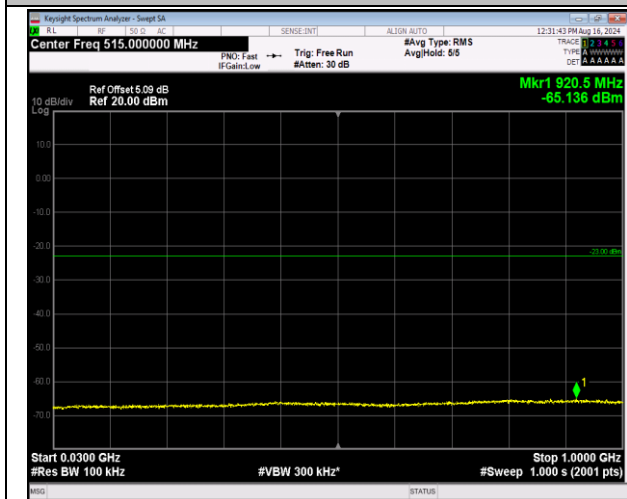
66-66-5MHz-20MHz-64QAM-64QAM-132330-132447-1R B#0-1RB#99-30~1000MHz-PASS
