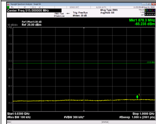
66-66-5MHz-20MHz-QPSK-QPSK-132455-132572-25RB #0-100RB#0-30~1000MHz-PASS
