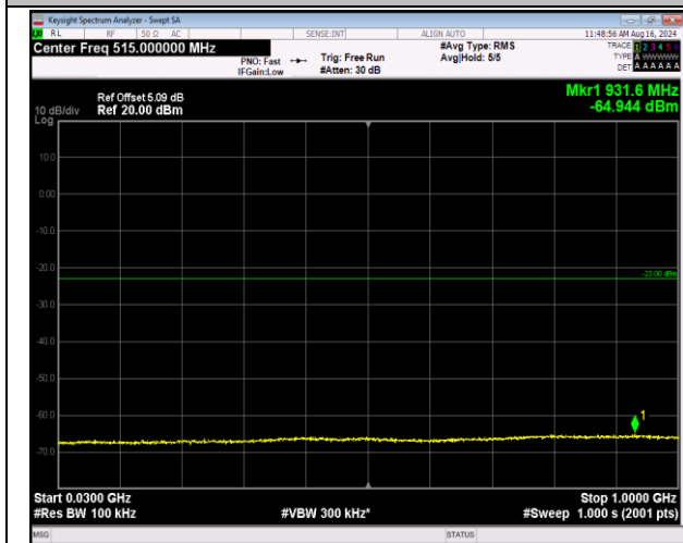
66-66-5MHz-20MHz-QPSK-QPSK-132330-132447-25RB #0-100RB#0-30-1000MHz-PASS
