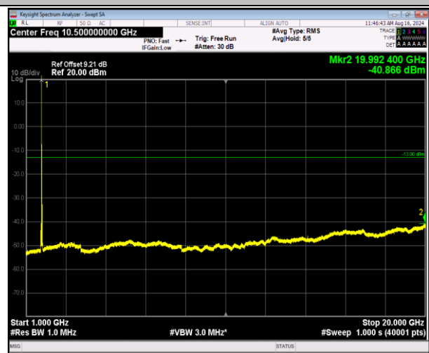
66-66-5MHz-20MHz-QPSK-QPSK-132330-132447-1RB#24 -0RB#0-1000-20000MHz-PASS
