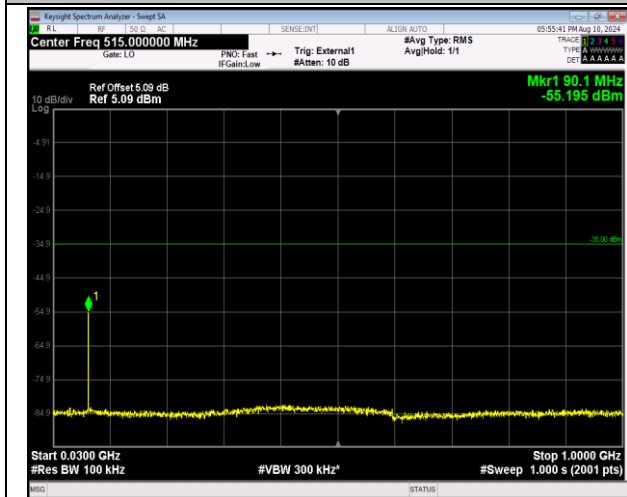
41-41-20MHz-20MHz-QPSK-QPSK-41292-41490-1RB#0 -0RB#0-30~1000MHz-PASS
