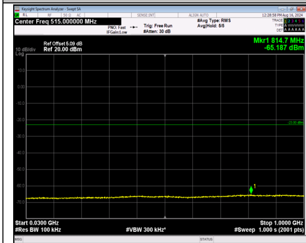
66-66-5MHz-20MHz-64QAM-64QAM-132005-132122-1R B#0-1RB#99-30~1000MHz-PASS
