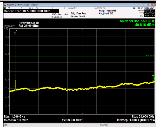
66-66-5MHz-20MHz-QPSK-QPSK-132005-132122-25RB#0 -100RB#0-1000~20000MHz-PASS
