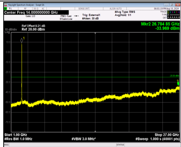
41-41-20MHz-20MHz-QPSK-QPSK-41292-41490-100RB#0 -100RB#0-1000~27000MHz-PASS
