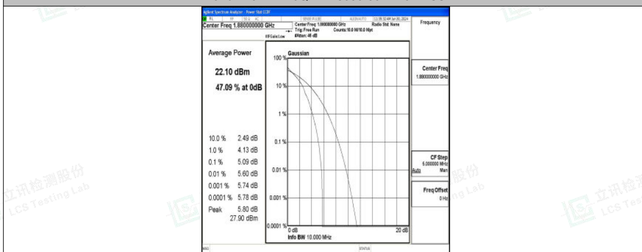
Band2-10MHz-QPSK-18900-1RB#0-PASS
