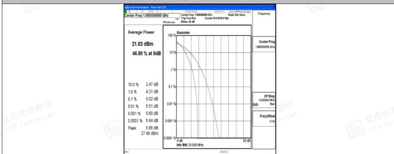
Band2-20MHz-QPSK-18900-1RB#0-PASS
