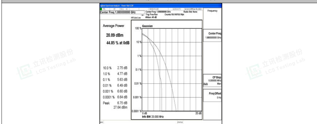
Band2-20MHz-16QAM-18900-1RB#0-PASS
