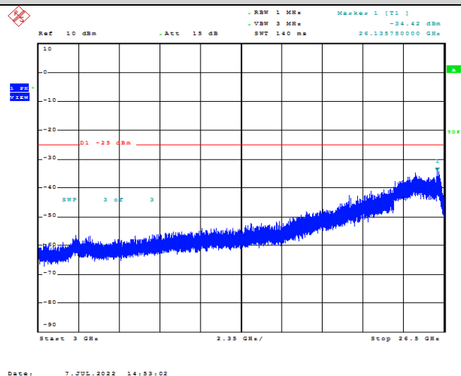
Band7-20MHz-QPSK-21350-1RB#0-Range1:3000~26500MHz
