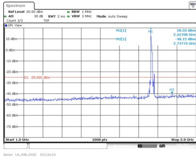
Band7-20MHz-QPSK-21100-1RB#0-Range2:1000~3000MHz
