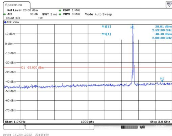
Band7-10MHz-QPSK-21100-1RB#0-Range2:1000~3000MHz
