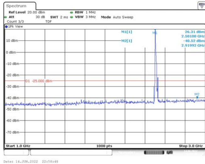
Band7-15MHz-QPSK-20825-1RB#0-Range2:1000~3000MHz
