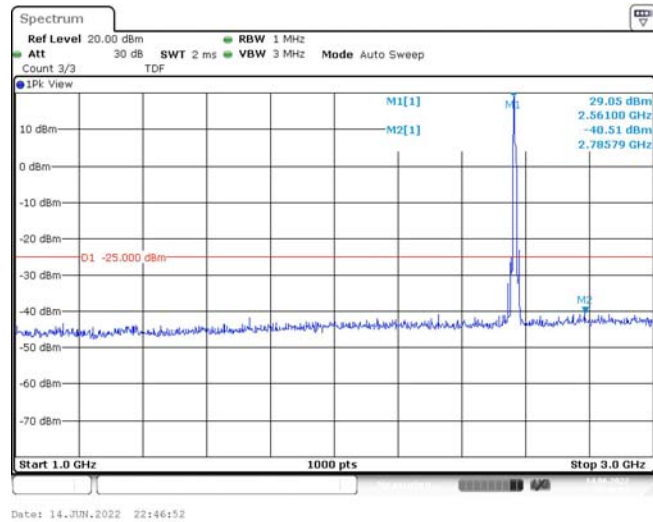
Band7-10MHz-QPSK-21400-1RB#0-Range2:1000~3000MHz
