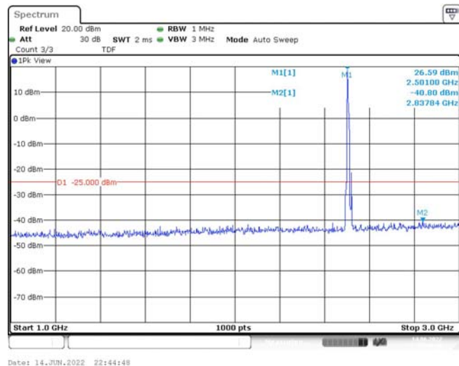
Band7-10MHz-QPSK-20800-1RB#0-Range2:1000~3000MHz
