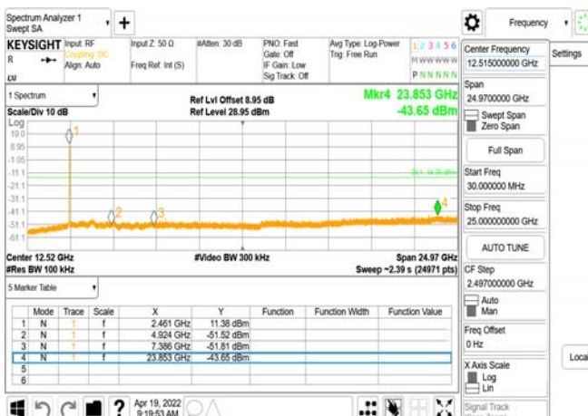
802.11ax_20MHz_Chain0_2462MHz
