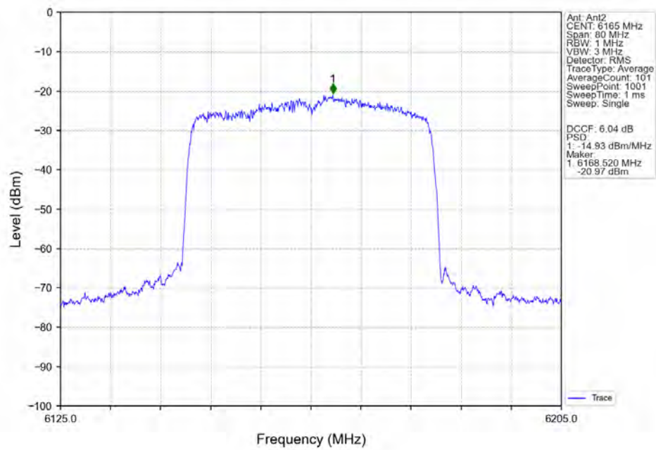
802.11ax(HEW40) MCH 6165MHz RU484 Left Ant2 NTNV
