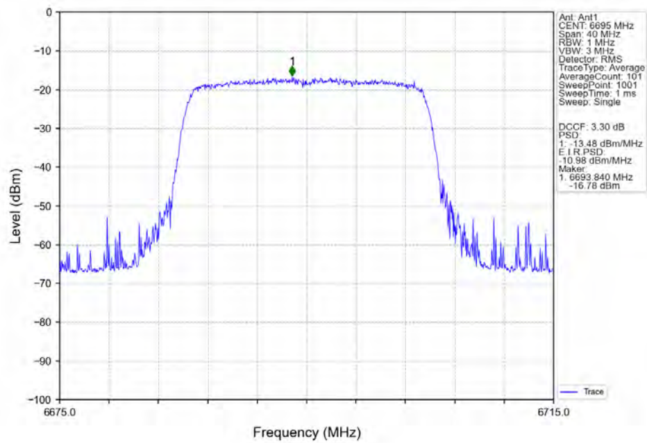
802.11ax(HEW20) MCH 6695MHz RU242 Left Ant1 NTN
