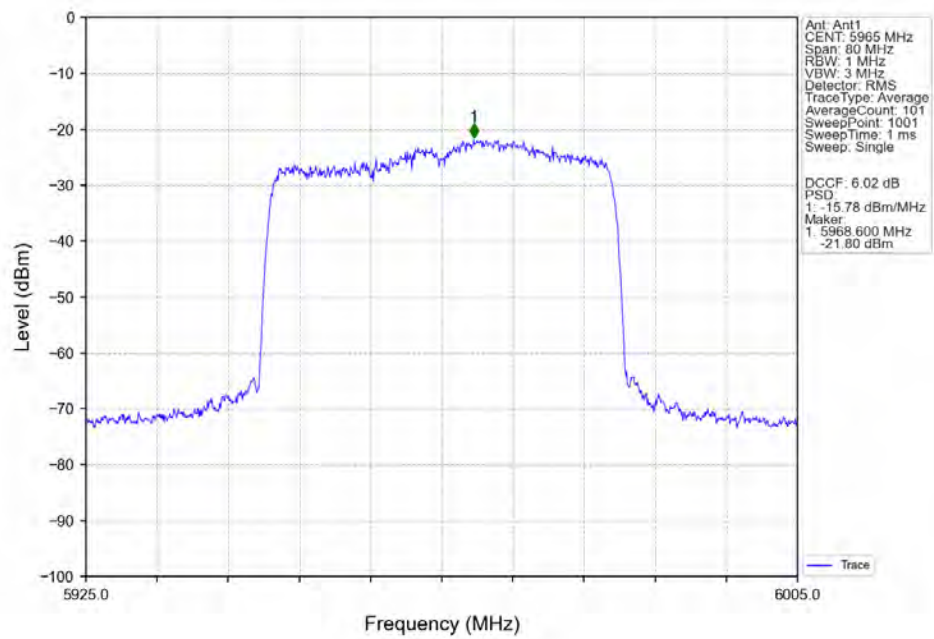
802.11ax(HEW40) LCH 5965MHz RU484 Left Ant1 NTN
