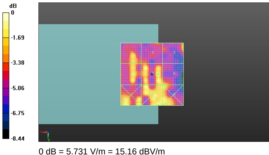
Fig A.4 HAC RF E-Field CDMA BC1
