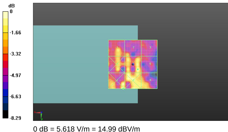
Fig A.5 HAC RF E-Field CDMA BC1
