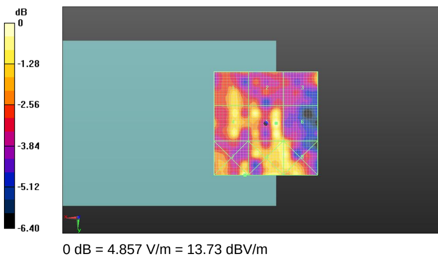
Fig A.6 HAC RF E-Field CDMA BC1
