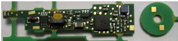
PCBA Type 2 top
