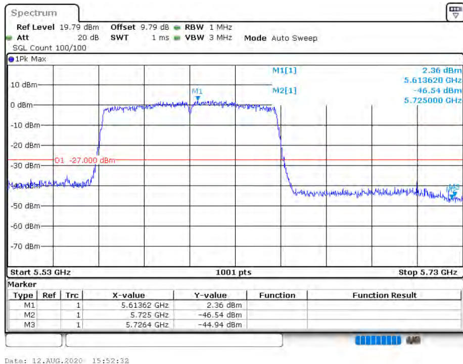
Band Edge NVNT 802.11ac80 5610MHz High Ant 1
