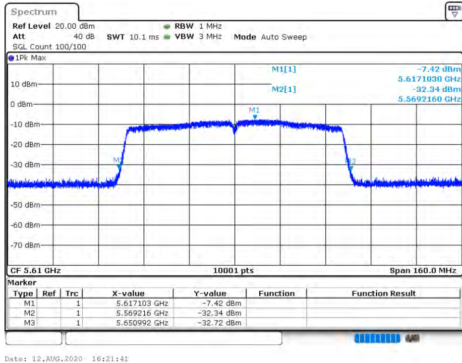
-26 dB BW NVNT 802.11ac80 5610MHz Ant 2
