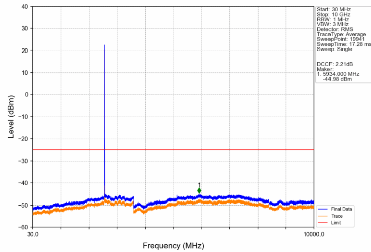
Band38 5MHz QPSK LCH 2572.5MHz RB 1 0 NTNV
