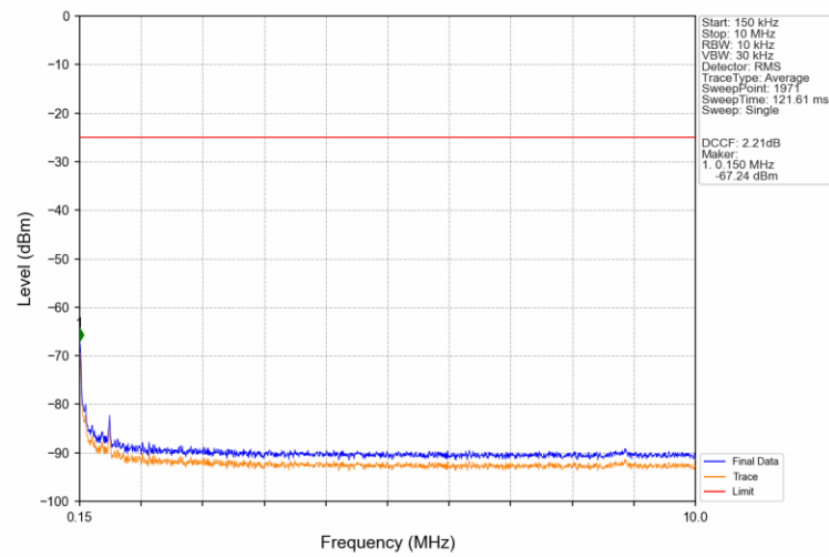
Band38_10MHz_QPSK_MCH_2595MHz_RB_1_0_NTNV
