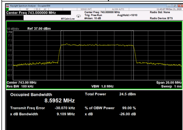
Figure 316: 64QAM 10MHz B.W.; 743.0MHz, 30kHz - Output
