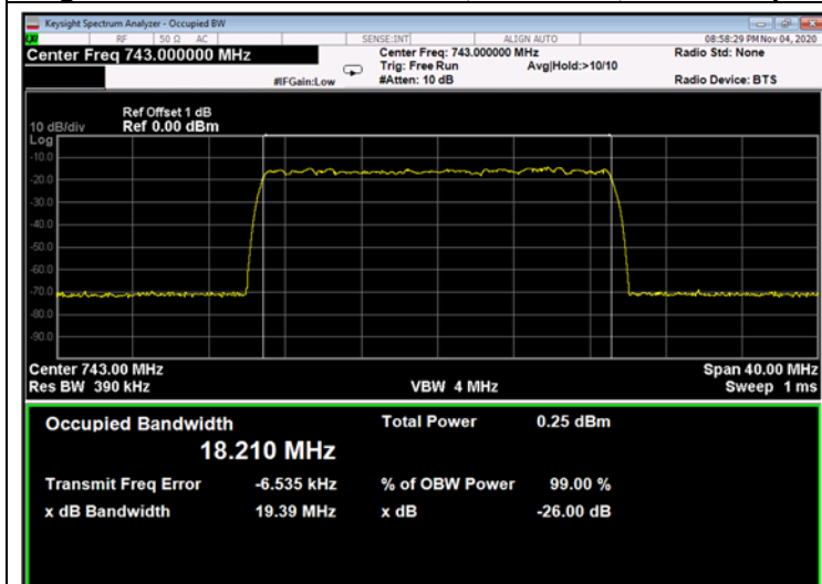
Figure 268: QPSK 20MHz B.W.; 743.0MHz, 30kHz - Input
