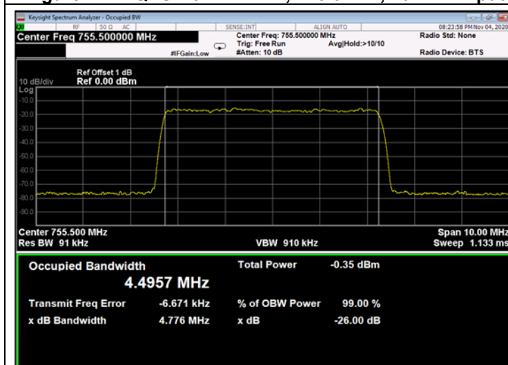
Figure 244: QPSK 5MHz B.W.; 755.5MHz, 15kHz - Input
