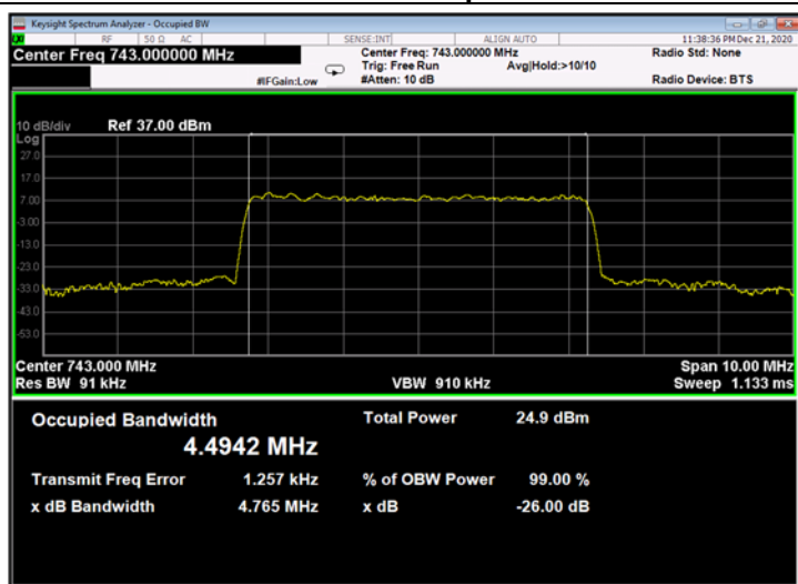
Figure 308: 64QAM 5MHz B.W.; 743.0MHz, 15kHz - Output
