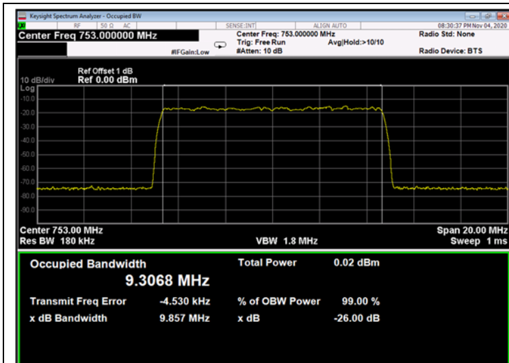
Figure 252: QPSK 10MHz B.W.; 753.0MHz, 15kHz - Input
