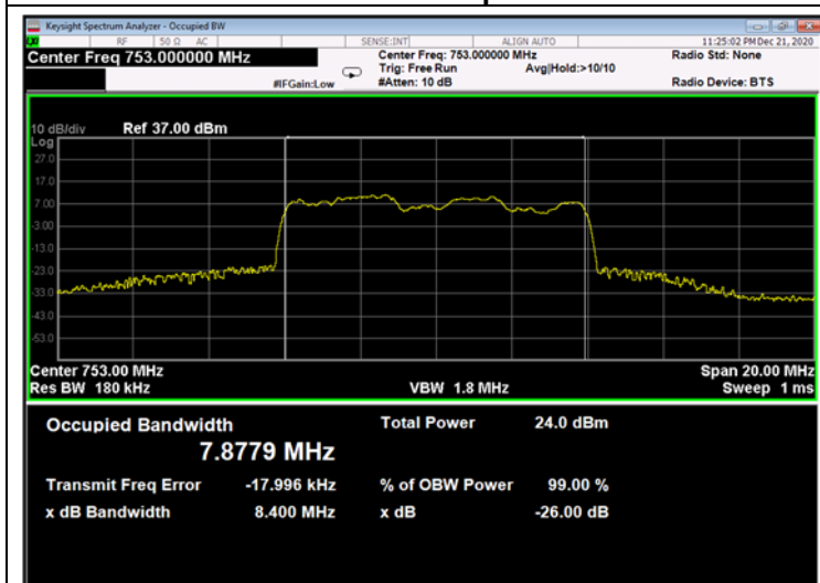
Figure 287: 16QAM 10MHz B.W.; 753.0MHz, 60kHz - Output
