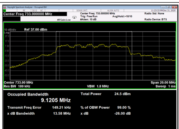
Figure 280: 16QAM 10MHz B.W.; 733.0MHz, 30kHz- Output
