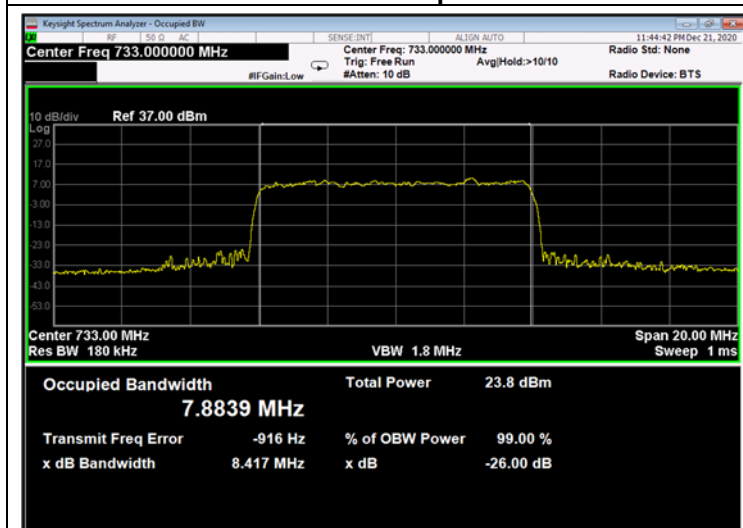
Figure 314: 64QAM 10MHz B.W.; 733.0MHz, 60kHz - Output
