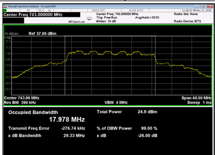
Figure 302: 16QAM 20MHz B.W.; 743.0MHz, 60kHz - Output
