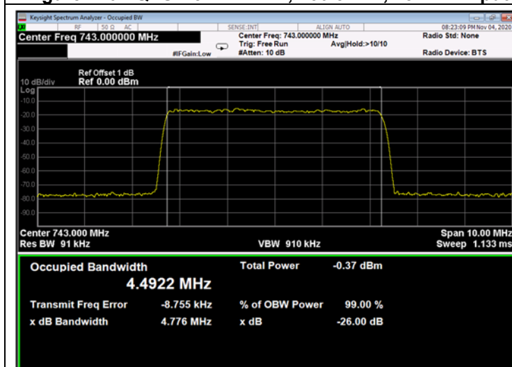
Figure 242: QPSK 5MHz B.W.; 743.0MHz, 15kHz - Input
