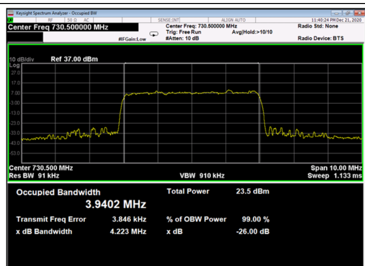
Figure 307: 64QAM 5MHz B.W.; 730.5MHz, 30kHz - Output
