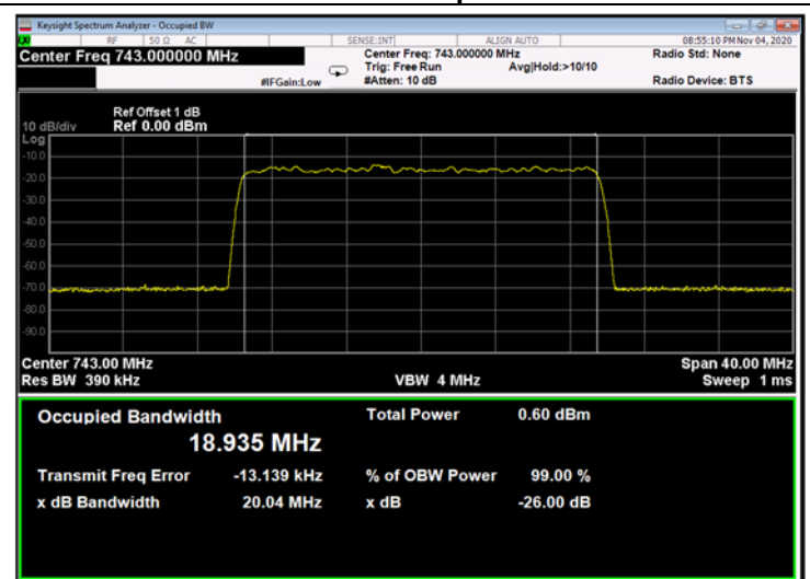
Figure 267: QPSK 20MHz B.W.; 743.0MHz, 15kHz - Input
