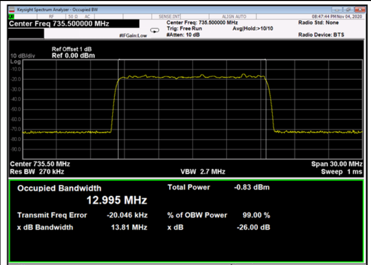
Figure 257: QPSK 15MHz B.W.; 735.5MHz, 60kHz - Input
