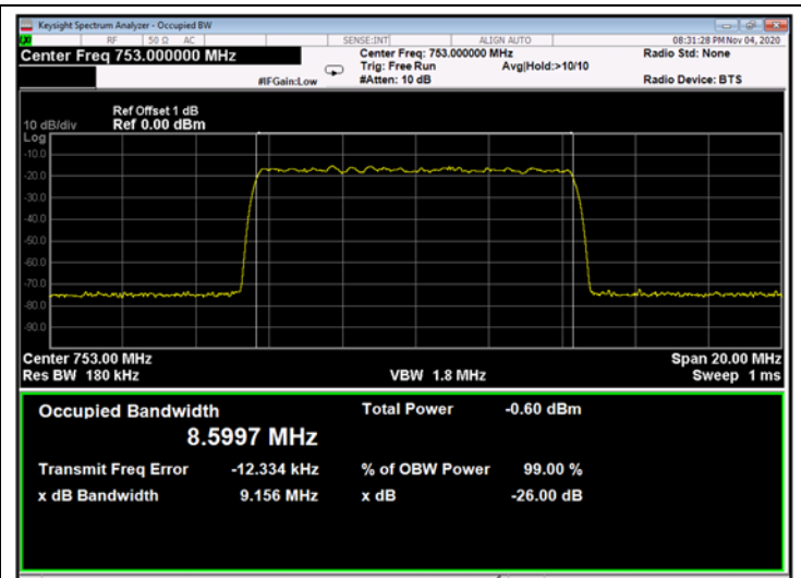
Figure 253: QPSK 10MHz B.W.; 753.0MHz, 30kHz - Input
