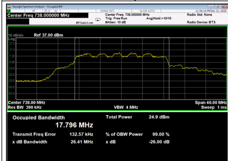
Figure 299: 16QAM 20MHz B.W.; 738.0MHz, 60kHz - Output
