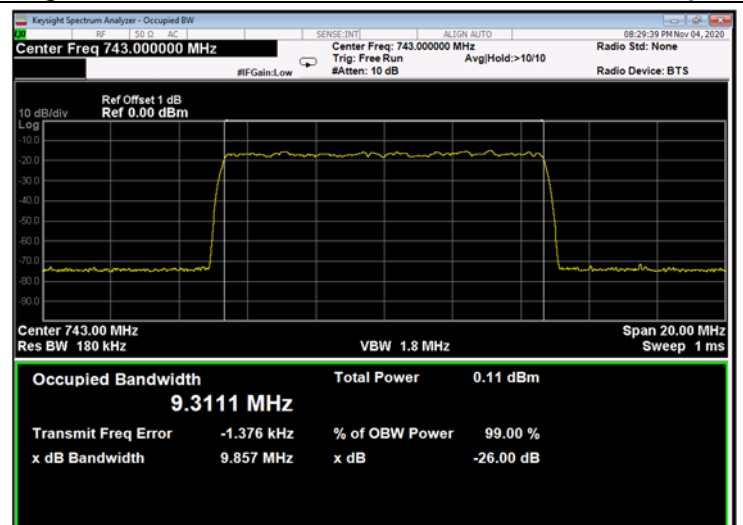
Figure 249: QPSK 10MHz B.W.; 743.0MHz, 15kHz - Input
