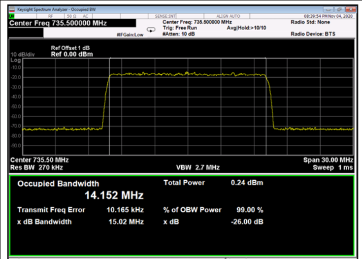
Figure 255: QPSK 15MHz B.W.; 735.5MHz, 15kHz - Input
