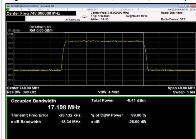
Figure 272: QPSK 20MHz B.W.; 748.0MHz, 60kHz - Input
