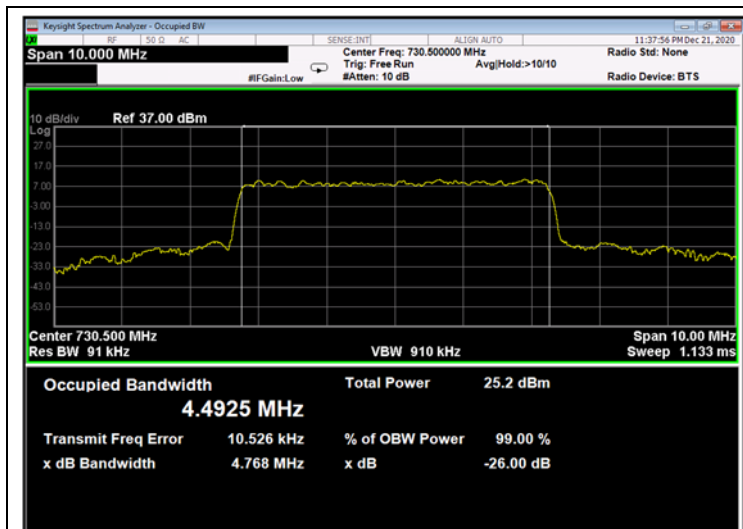
Figure 306: 64QAM 5MHz B.W.; 730.5MHz, 15kHz - Output
