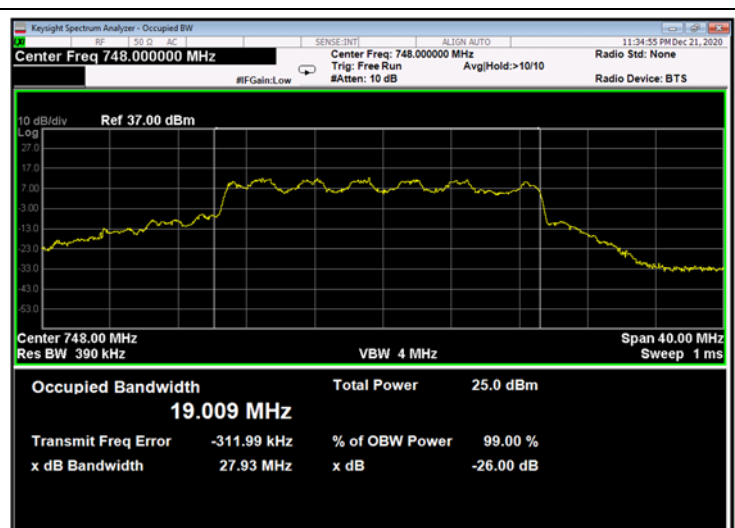
Figure 304: 16QAM 20MHz B.W.; 748.0MHz, 30kHz - Output
