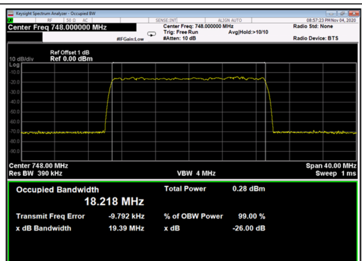
Figure 271: QPSK 20MHz B.W.; 748.0MHz, 30kHz - Input
