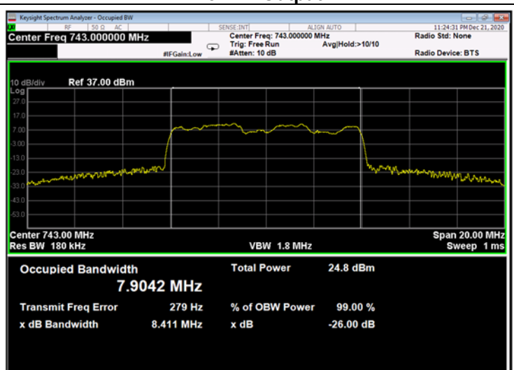
Figure 284: 16QAM 10MHz B.W.; 743.0MHz, 60kHz - Output
