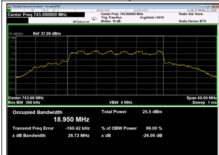
Figure 301: 16QAM 20MHz B.W.; 743.0MHz, 30kHz - Output
