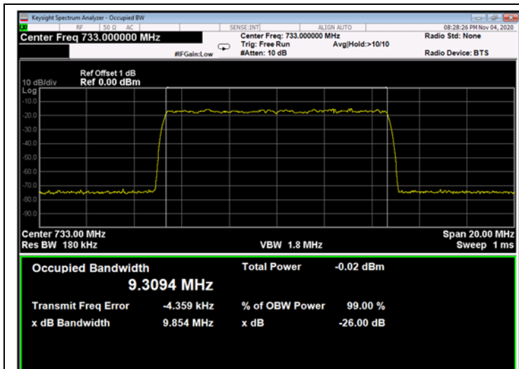
Figure 246: QPSK 10MHz B.W.; 733.0MHz, 15kHz - Input
