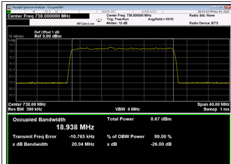
Figure 264: QPSK 20MHz B.W.; 738.0MHz, 15kHz - Input
