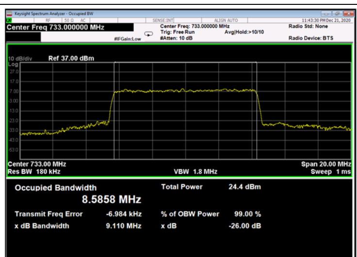
Figure 313: 64QAM 10MHz B.W.; 733.0MHz, 30kHz - Output
