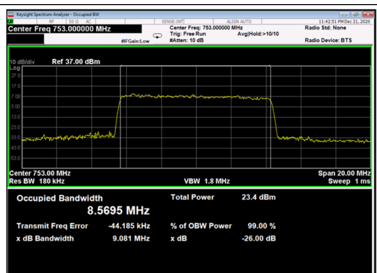
Figure 319: 64QAM 10MHz B.W.; 753.0MHz, 30kHz - Output
