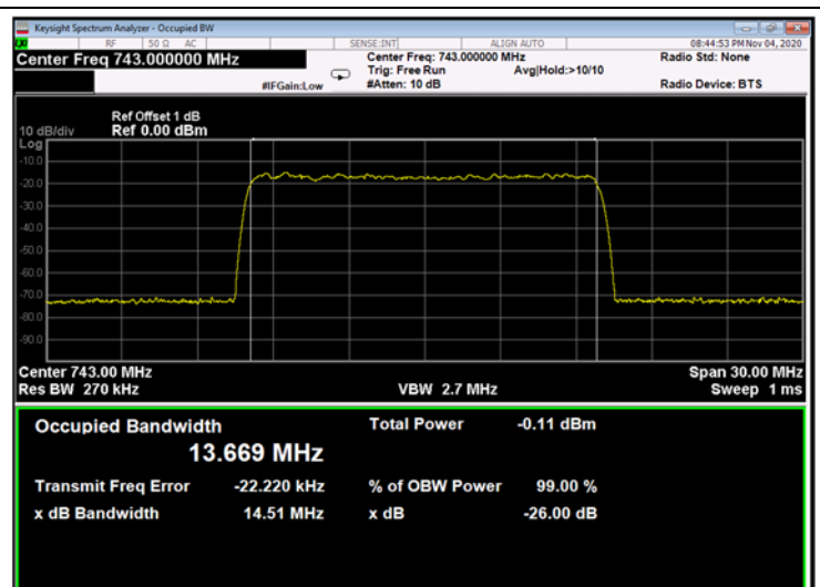
Figure 259: QPSK 15MHz B.W.; 743.0MHz, 30kHz - Input
