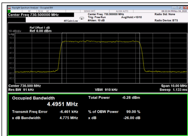
Figure 240: QPSK 5MHz B.W.; 730.5MHz, 15kHz - Input
