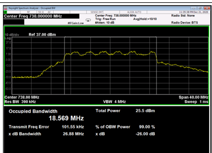
Figure 298: 16QAM 20MHz B.W.; 738.0MHz, 30kHz - Output
