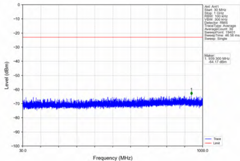
n66_30kHz_SISO_NTNV_20MHz_DFT-s-OFDM_QPSK_1770MHz_Inner_1RB_Right
