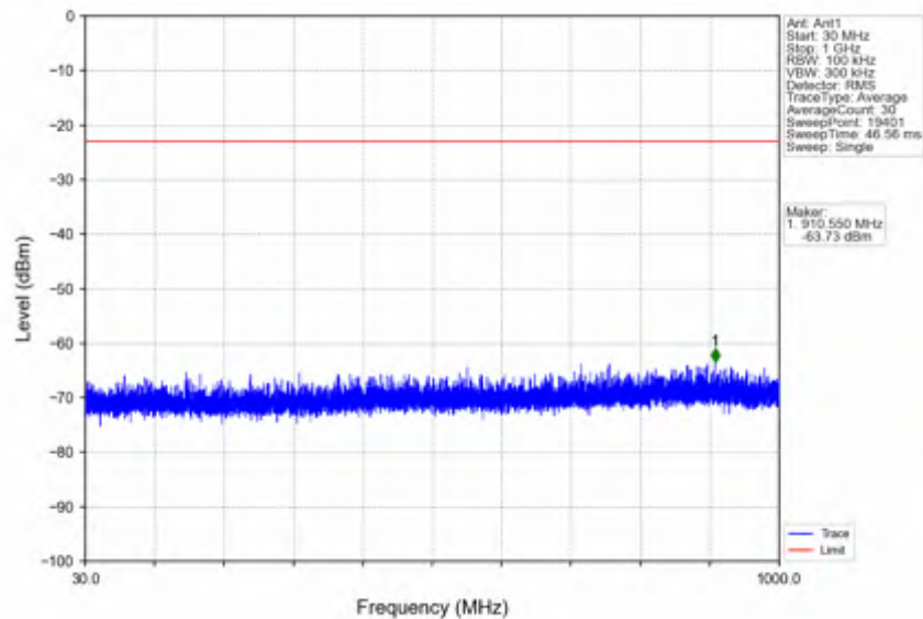
n66_30kHz_SISO_NTNV_20MHz_CP-OFDM_QPSK_1720MHz_Edge_1RB_Left
