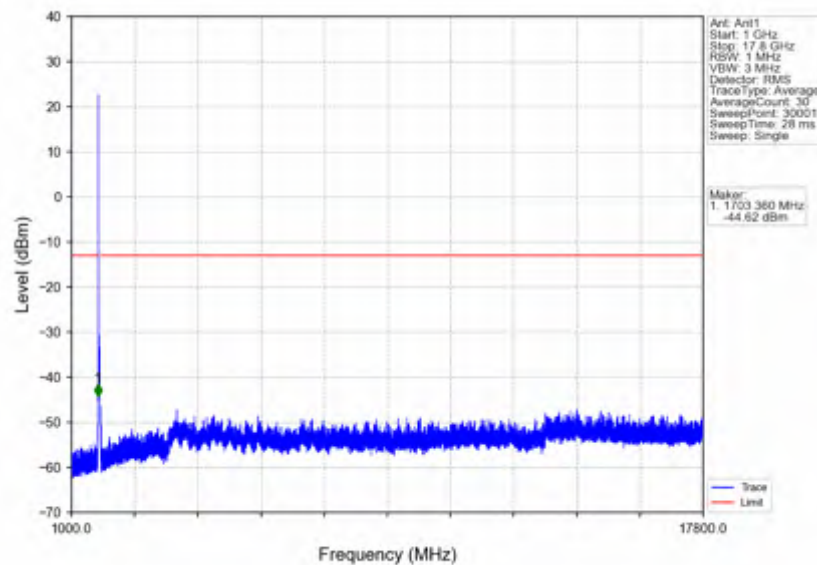
n66_30kHz_SISO_NTNV_40MHz_DFT-s-OFDM_QPSK_1730MHz_Inner_1RB_Left
