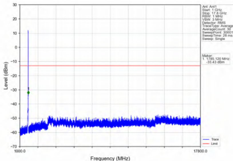
n66_30kHz_SISO_NTNV_20MHz_DFT-s-OFDM QPSK_1770MHz_Inner_1RB_Right
