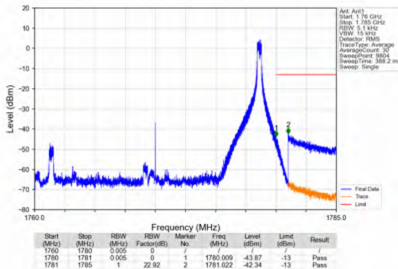
n66_30kHz_SISO_NTNV_20MHz_DFT-s-OFDM QPSK_1770MHz_Inner_1RB_Right
