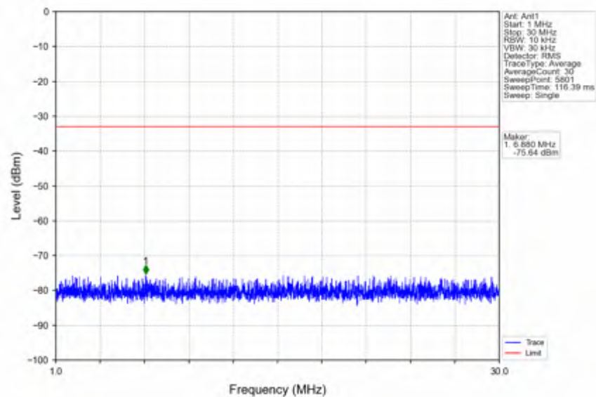
n66 30kHz SISO NTVN 20MHz DFT-s-OFDM QPSK 1770MHz Edge 1RB Right
