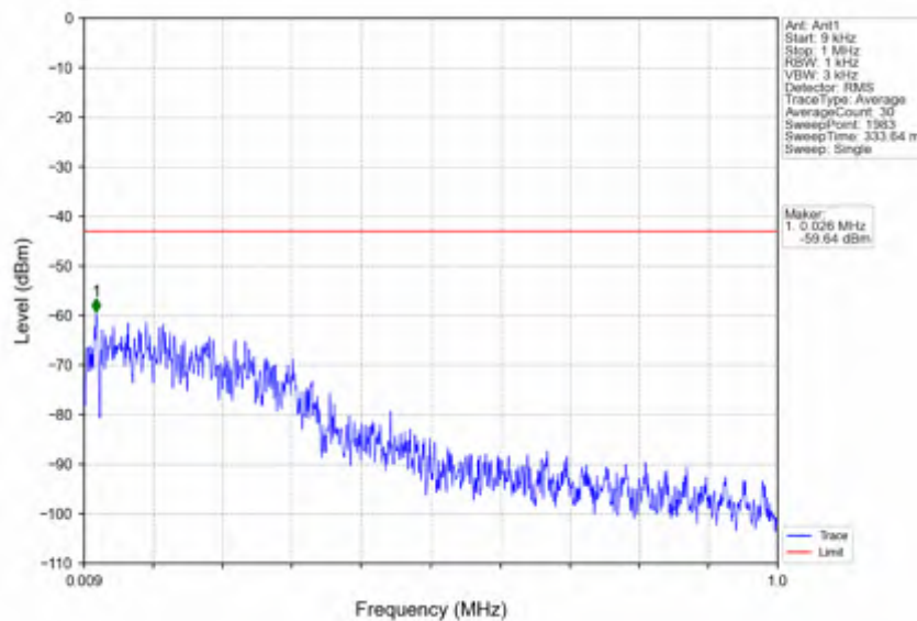
n66_30kHz_SISO_NTV_25MHz_CP-OFDM_QPSK_1722.5MHz_Inner_1RB_Left
