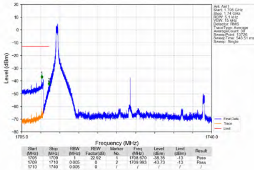
n66_30kHz_SISO_NTNV_30MHz_DFT-s-OFDM QPSK_1725MHz_Inner_1RB_Left
