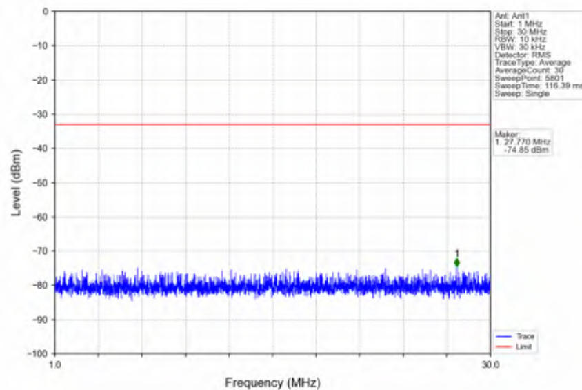
n66_30kHz_SISO_NTNV_20MHz_CP-OFDM_QPSK_1720MHz_Inner_1RB_Left
