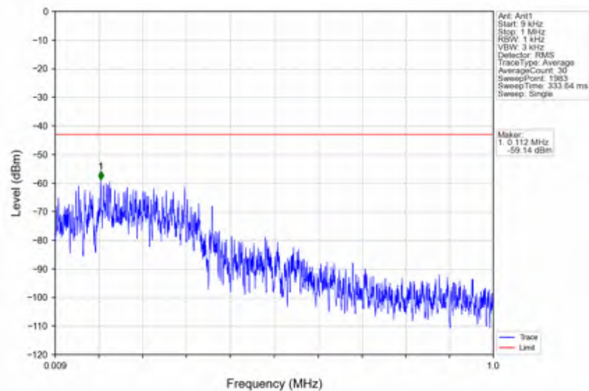
n66_30kHz_SISO_NTNV_30MHz_DFT-s-OFDM QPSK_1765MHz_Inner_1RB_Right
