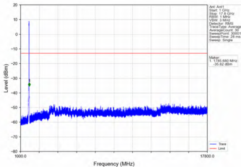
n66_30kHz_SISO_NTNV_40MHz_DFT-s-OFDM QPSK_1760MHz_Inner_1RB_Right
