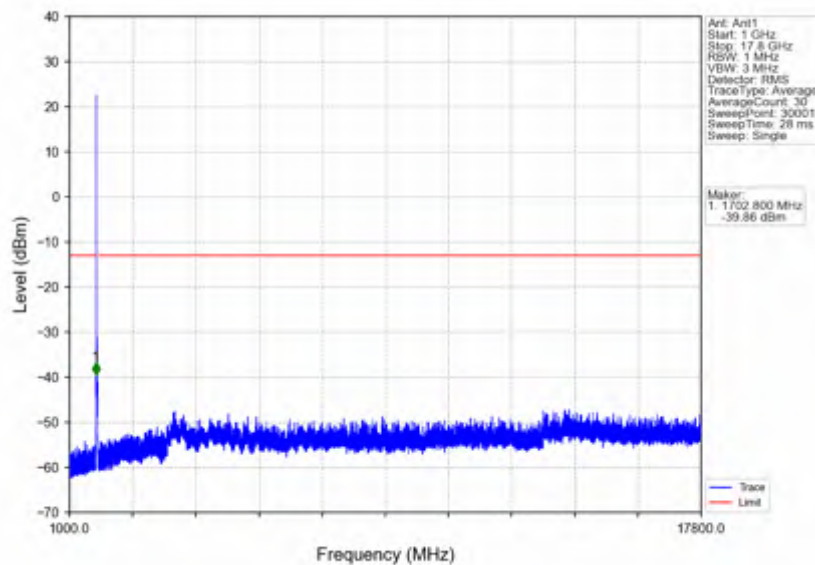
n66_30kHz_SISO_NTNV_20MHz_DFT-s-OFDM_QPSK_1720MHz_Inner_1RB_Left
