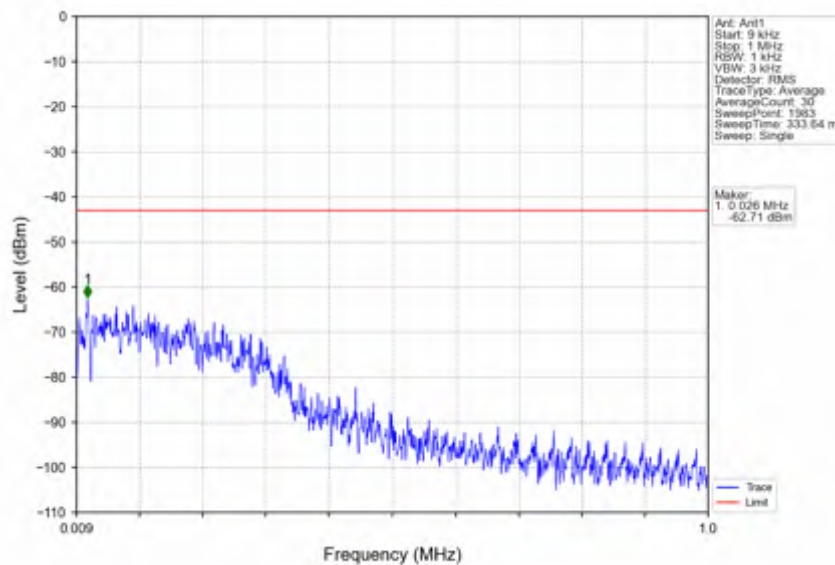
n66_30kHz_SISO_NTNV_20MHz_CP-OFDM_QPSK_1720MHz_Edge_1RB_Left
