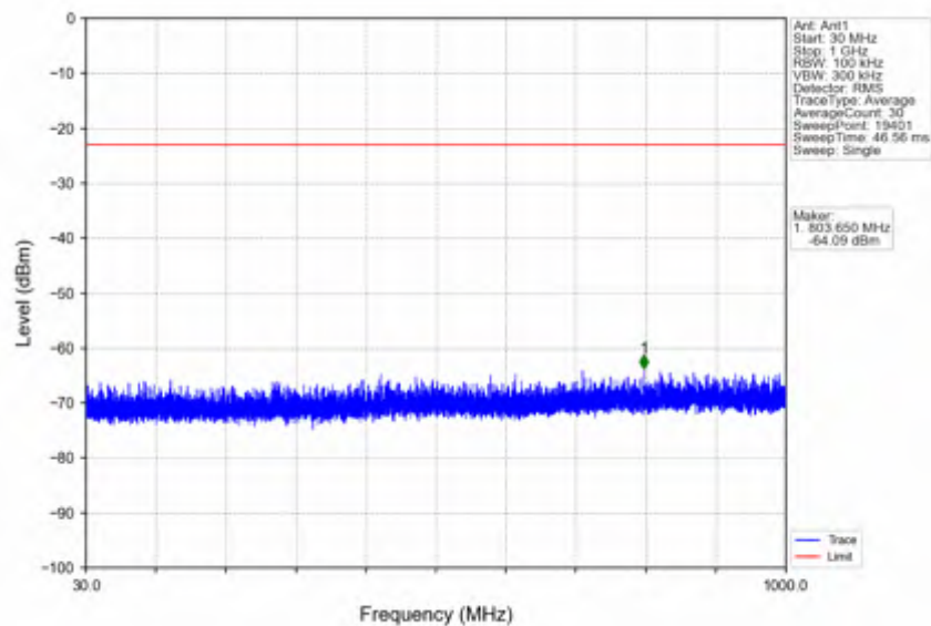
n66_30kHz_SISO_NTNV_30MHz_DFT-s-OFDM QPSK_1765MHz_Inner_1RB_Right
