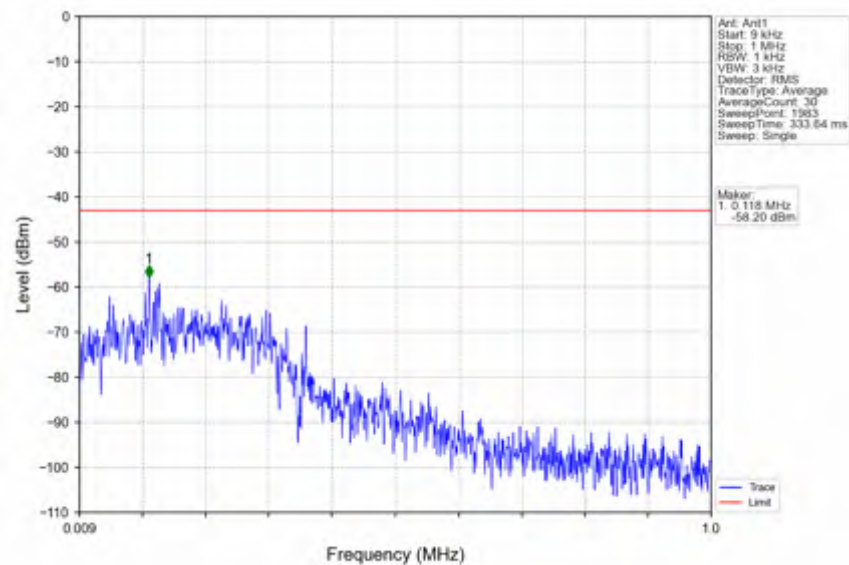
n66_30kHz_SISO_NTNV_20MHz_DFT-s-OFDM QPSK_1770MHz_Inner_1RB_Right
