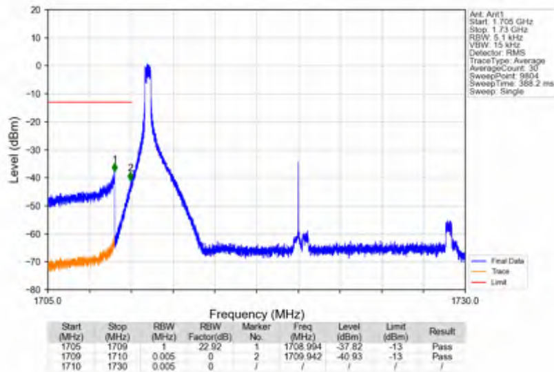
n66_30kHz_SISO_NTNV_20MHz_CP-OFDM_QPSK_1720MHz_Edge_1RB_Left
