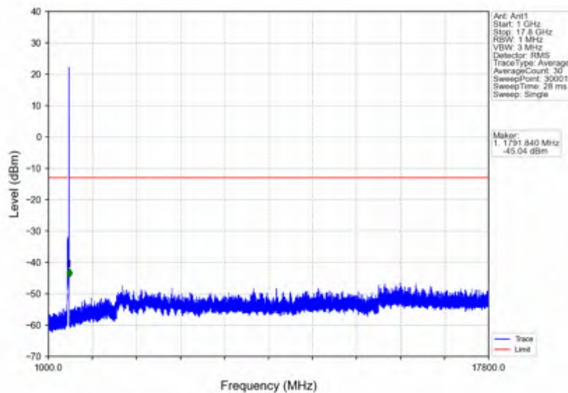
n66_30kHz_SISO_NTNV_30MHz_DFT-s-OFDM QPSK_1765MHz_Inner_1RB_Right
