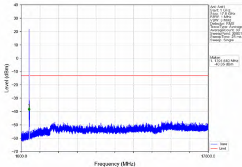
n66_30kHz_SISO_NTNV_20MHz_DFT-s-OFDM QPSK_1720MHz_Edge_1RB_Left
