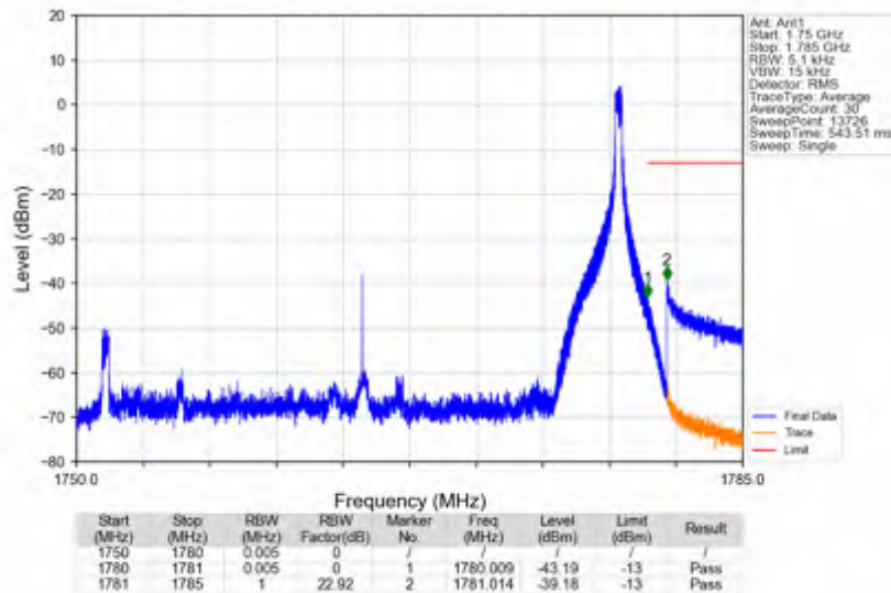
n66_30kHz_SISO_NTNV_30MHz_DFT-s-OFDM QPSK_1765MHz_Inner_1RB_Right
