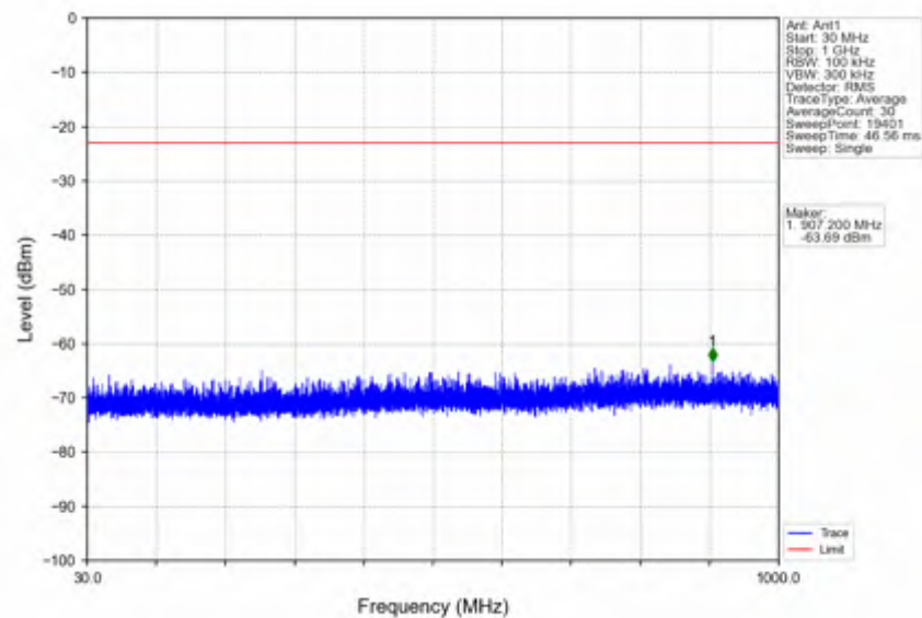
n66_30kHz_SISO_NTNV_40MHz_DFT-s-OFDM_QPSK_1730MHz_Inner_1RB_Left
