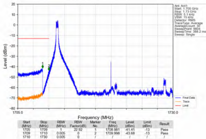
n66_30kHz_SISO_NTNV_20MHz_DFT-s-OFDM QPSK_1720MHz_Inner_1RB_Left
