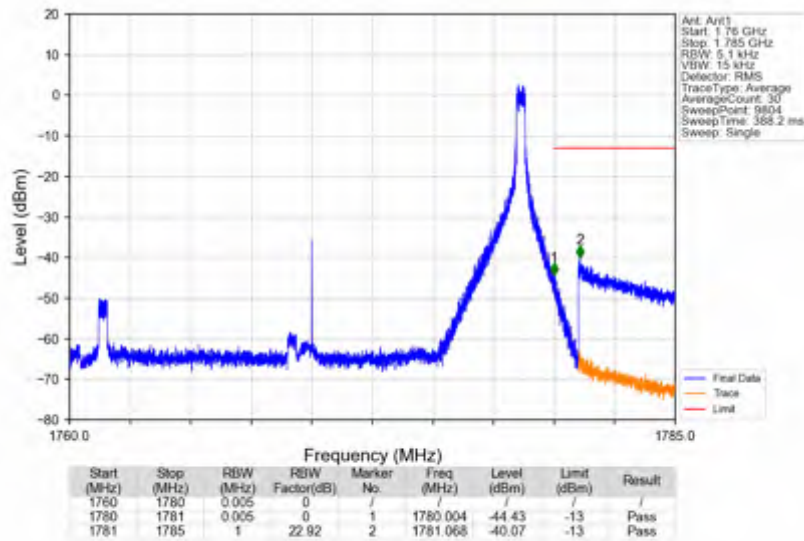
n66 30kHz SISO NTN 20MHz CP-OFDM QPSK 1770MHz Inner 1RB Right
