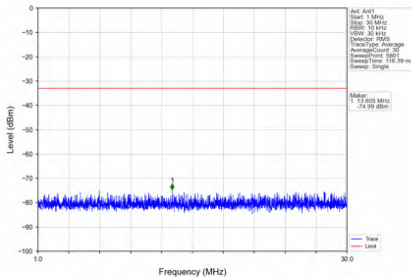
n66_30kHz_SISO_NTV_25MHz_CP-OFDM_QPSK_1722.5MHz_Inner_1RB_Left
