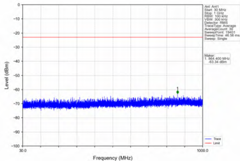
n66_30kHz_SISO_NTNV_20MHz_DFT-s-OFDM QPSK_1720MHz_Edge_1RB_Left
