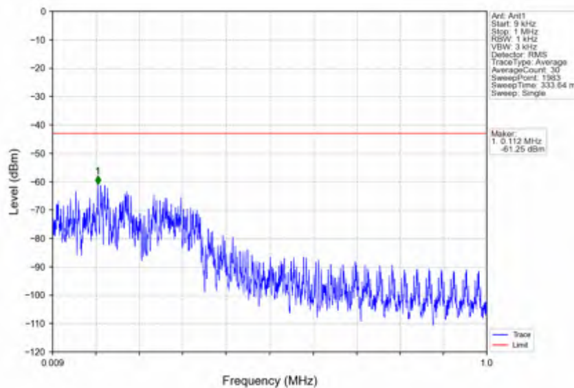
n66_30kHz_SISO_NTNV_30MHz_DFT-s-OFDM PI/2 BPSK_1725MHz_Inner_1RB_Left
