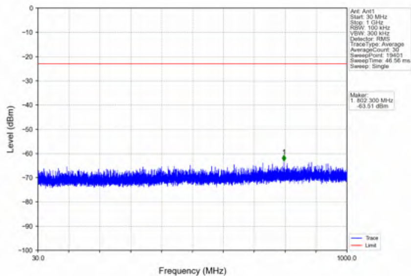
n66_30kHz_SISO_NTNV_20MHz_DFT-s-OFDM_QPSK_1720MHz_Inner_1RB_Left
