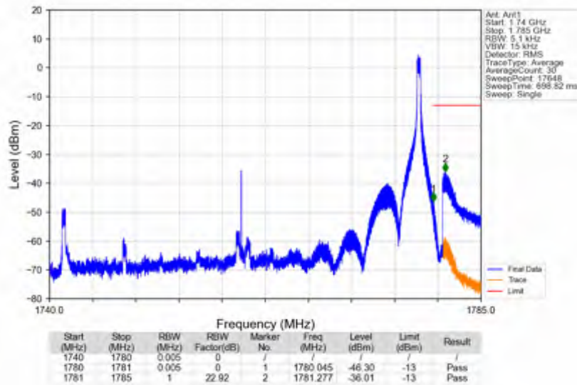
n66_30kHz_SISO_NTNV_40MHz_DFT-s-OFDM QPSK_1760MHz_Inner_1RB_Right
