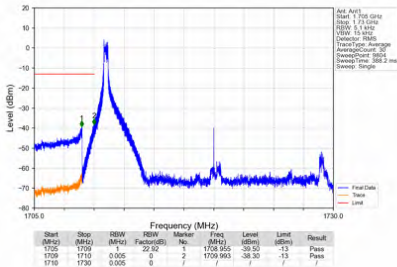
n66_30kHz_SISO_NTNV_20MHz_DFT-s-OFDM QPSK_1720MHz_Edge_1RB_Left
