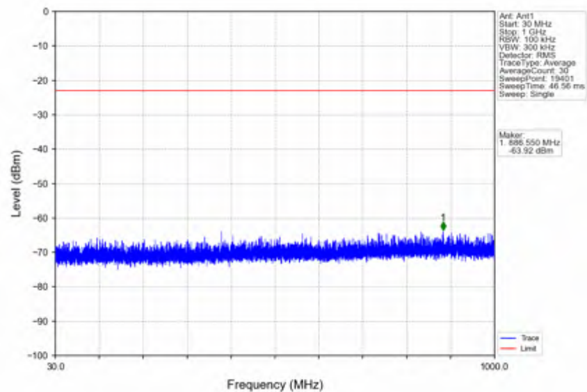
n66_30kHz_SISO_NTNV_20MHz_CP-OFDM QPSK_1770MHz_Inner_1RB_Right
