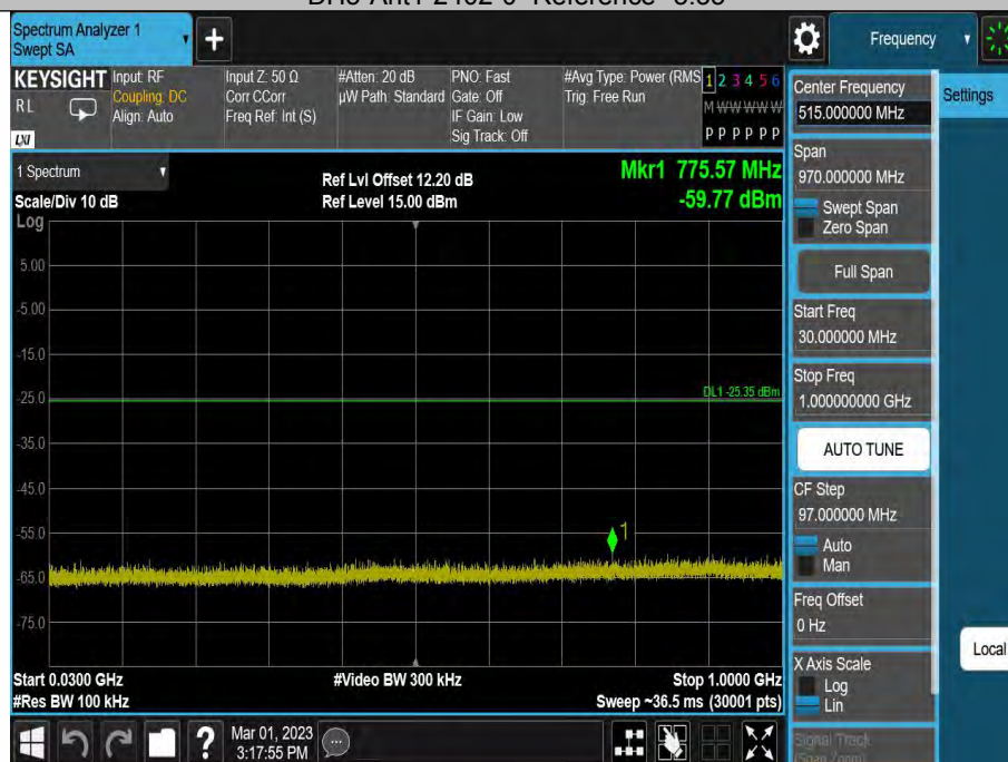
DH5-Ant1-2402-30~1000--5.35
