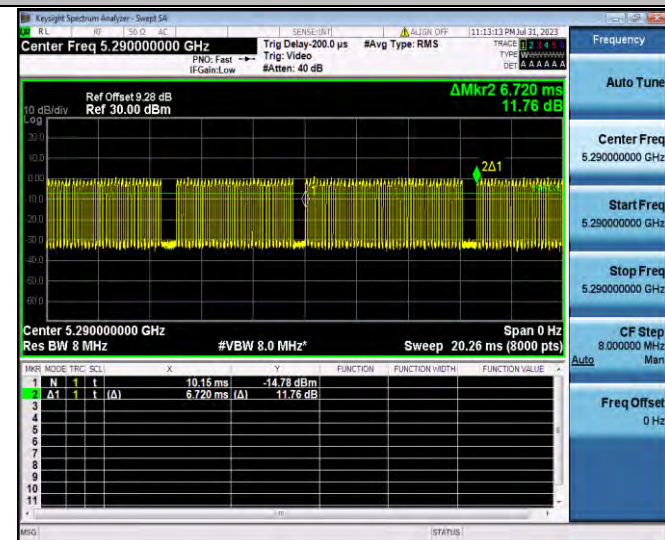
11AX80SISO_Ant1_5290
