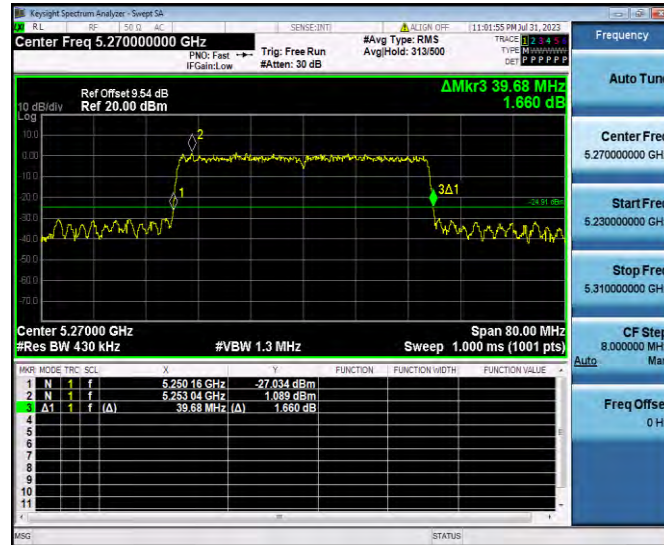
11AX40SISO_Ant1_5270
