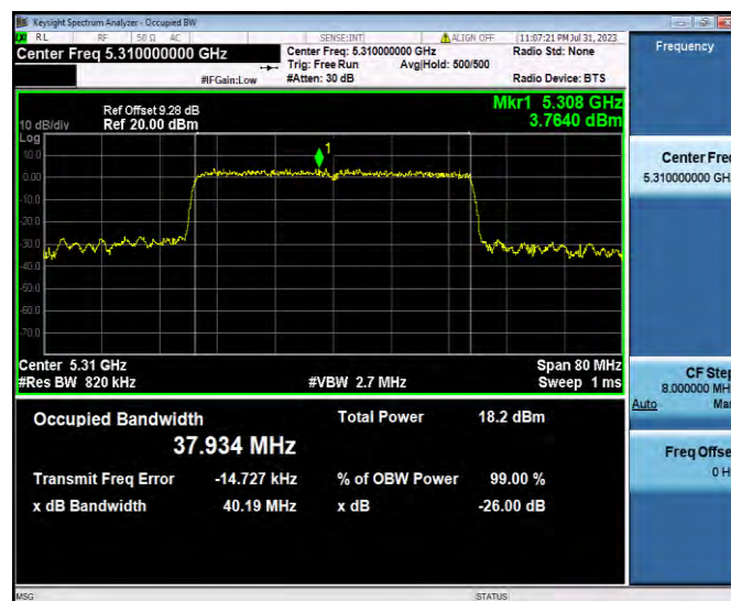
11AX40SISO_Ant1_5310
