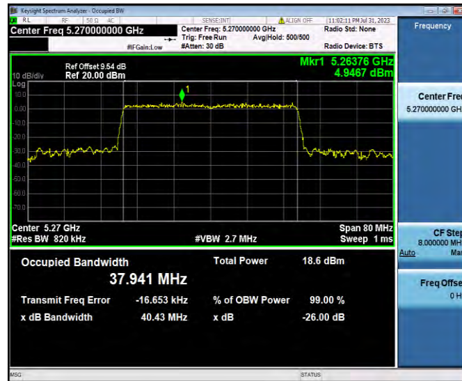
11AX40SISO_Ant1_5270
