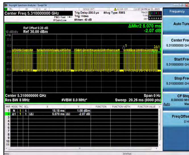
11AX40SISO_Ant1_5310
