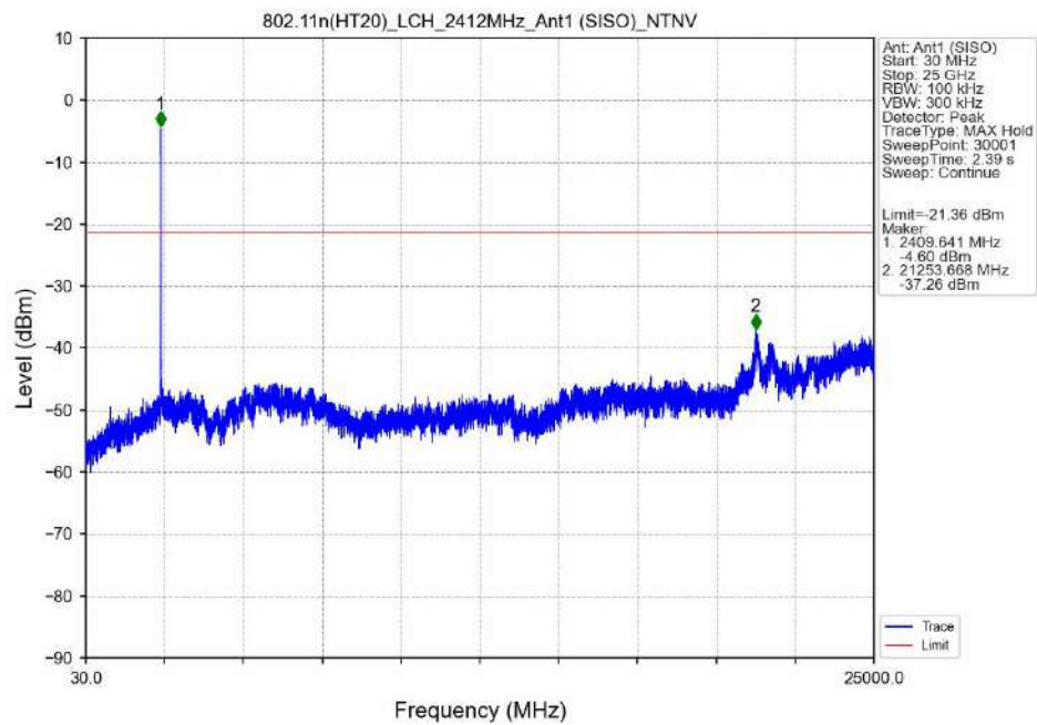
802.11n(HT20)_LCH_2412MHz_Ant1 (SISO)_NTNV
