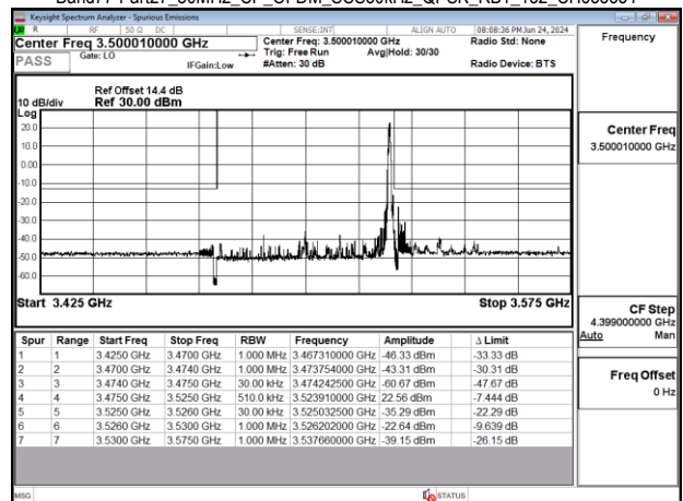
Band77-Part27_50MHz_CP_OFDM_SCS30kHz_QPSK_RB1_132_CH633334
