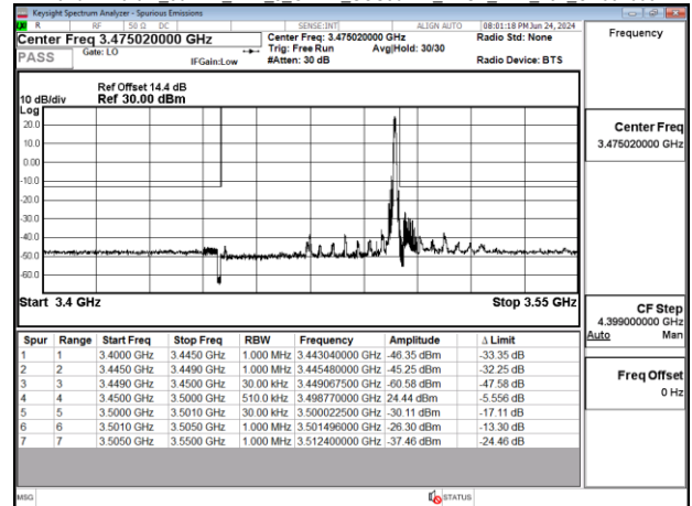
Band77-Part27_50MHz_DFT_s_OFDM_SCS30kHz_BPSK_RB1_132_CH633334
