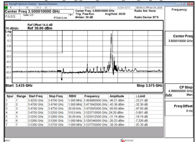
Band77-Part27_50MHz_DFT_s_OFDM_SCS30kHz_BPSK_RB1_132_CH633334
