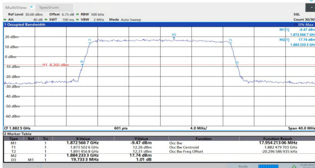
Band25-20MHz-QPSK-26365-100RB#0-PASS
