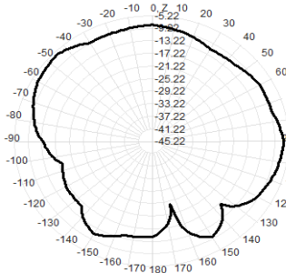
2480.0MHz Total(E1-XZ), Max= -6.29dBi
