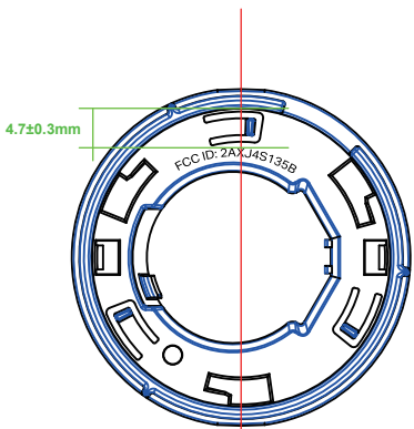
尺寸图
