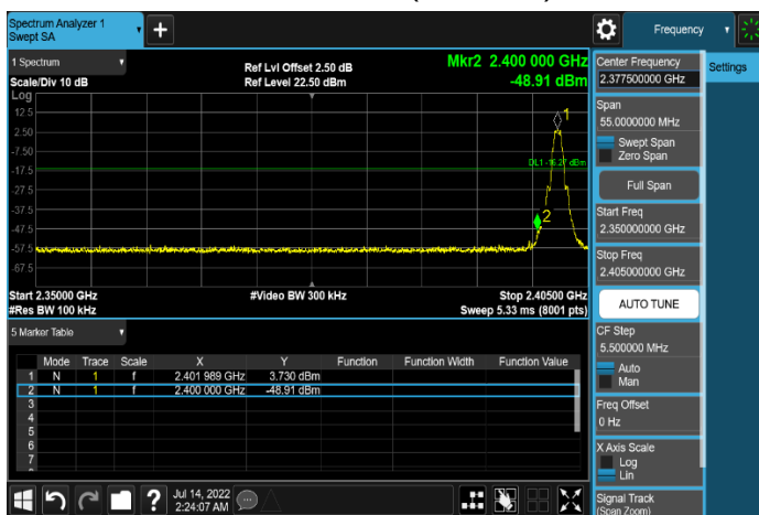
Mode 1 CH00 (2402MHz)
