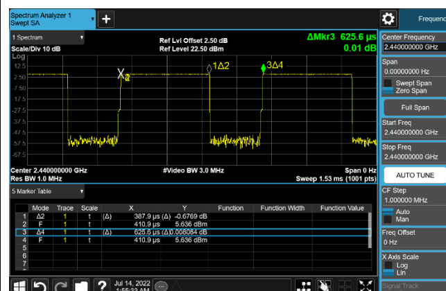
Mode 1 CH19 2440MHz
