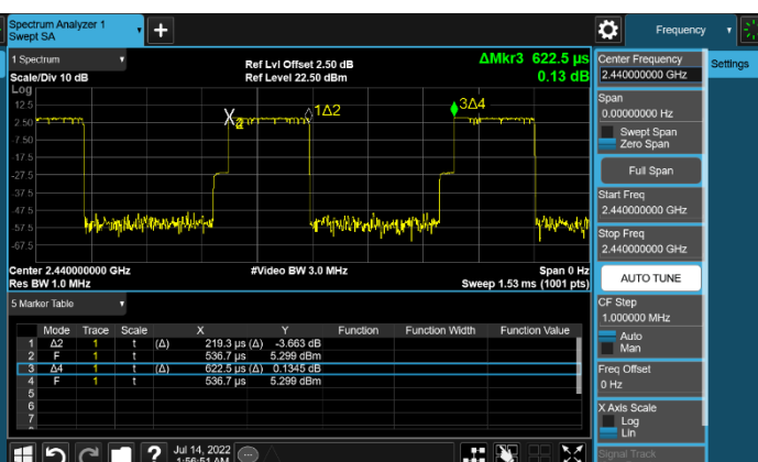
Mode 2 CH19 2440MHz
