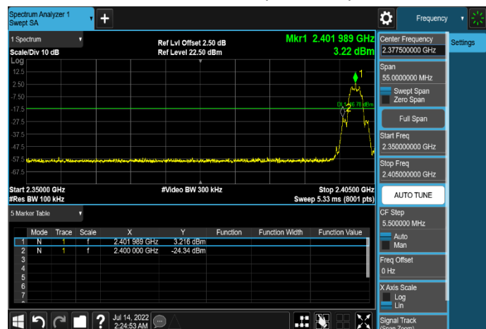
Mode 2 CH00 (2402MHz)
