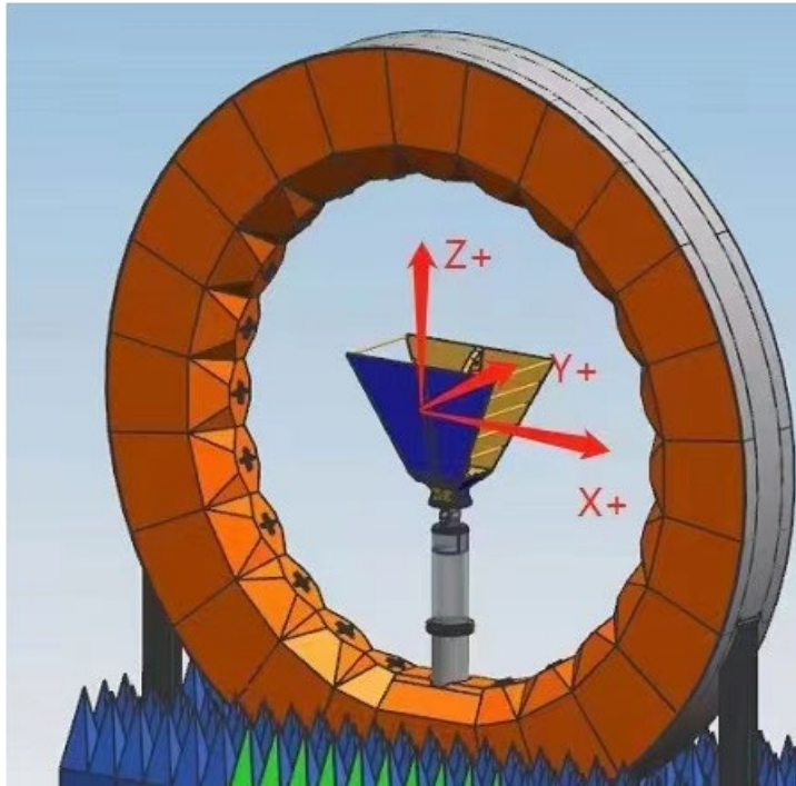
Primary antenna/RF1
