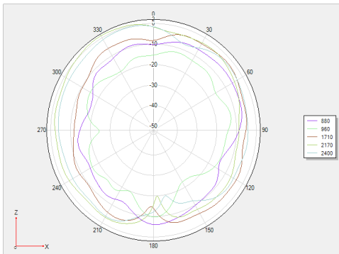
Primary antenna/RF1
