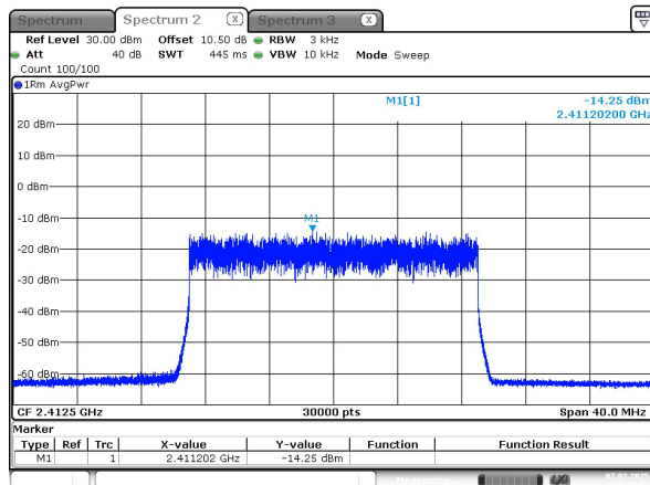
20M_2412.5 MHz_Chain 0
