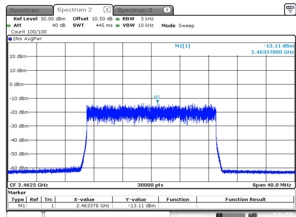
20M_2462.5 MHz_Chain 1
