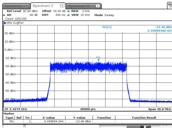
20M_2437.5 MHz_Chain 1
