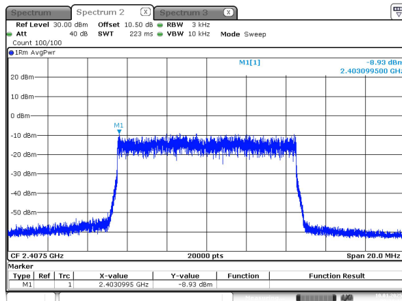
10M_2407.5 MHz_Chain 1
