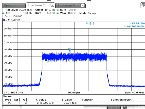
20M_2462.5 MHz_Chain 0
