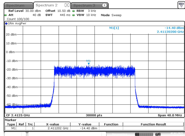
20M_2412.5 MHz_Chain 1
