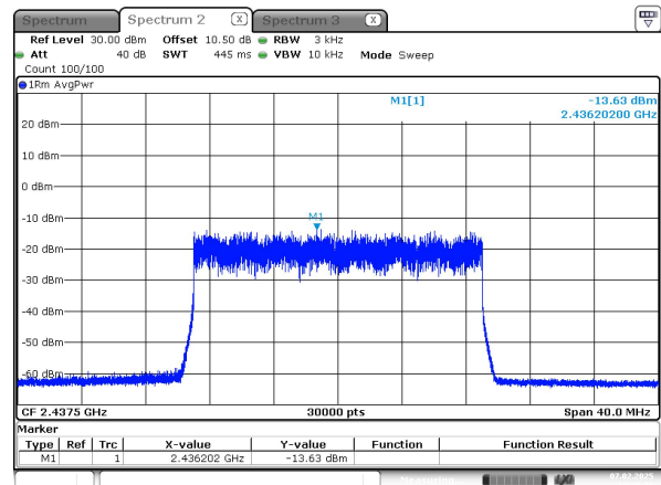
20M_2437.5 MHz_Chain 0
