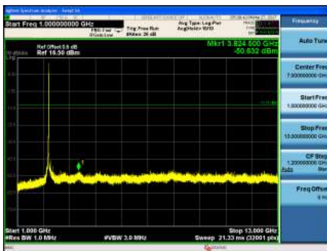
802.11b CH011 (2462MHz) -Ant 1
