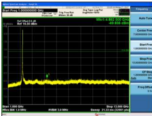
802.11g CH011 (2462MHz) -Ant 2
