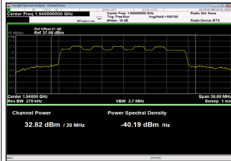
Figure 35: 16QAM 20MHz B.W.; 1940.0MHz, 60kHz
