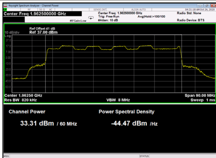
Figure 71: 16QAM 60MHz B.W.; 1962.5MHz, 30kHz
