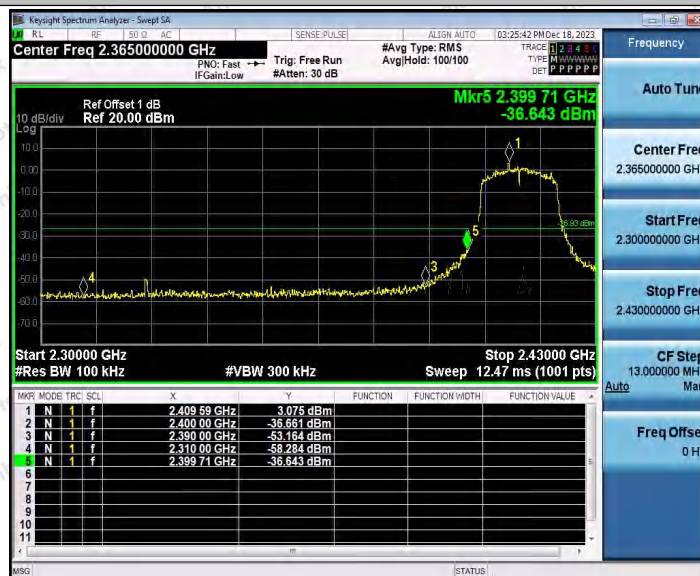
802.11n(HT20) SISO_Ant1_Low_2412
