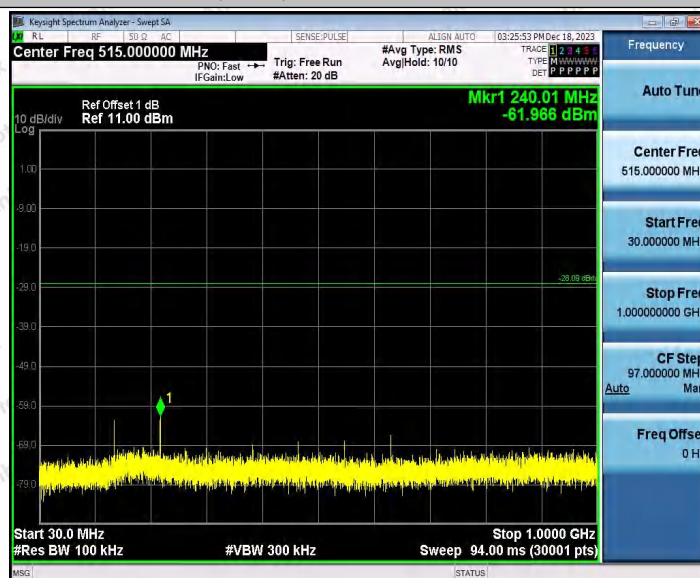
802.11n(HT20) SISO_Ant1_2412_30~1000
