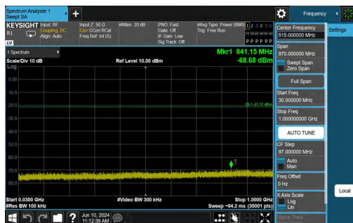
11G-Ant1-2412-30~1000-PASS
