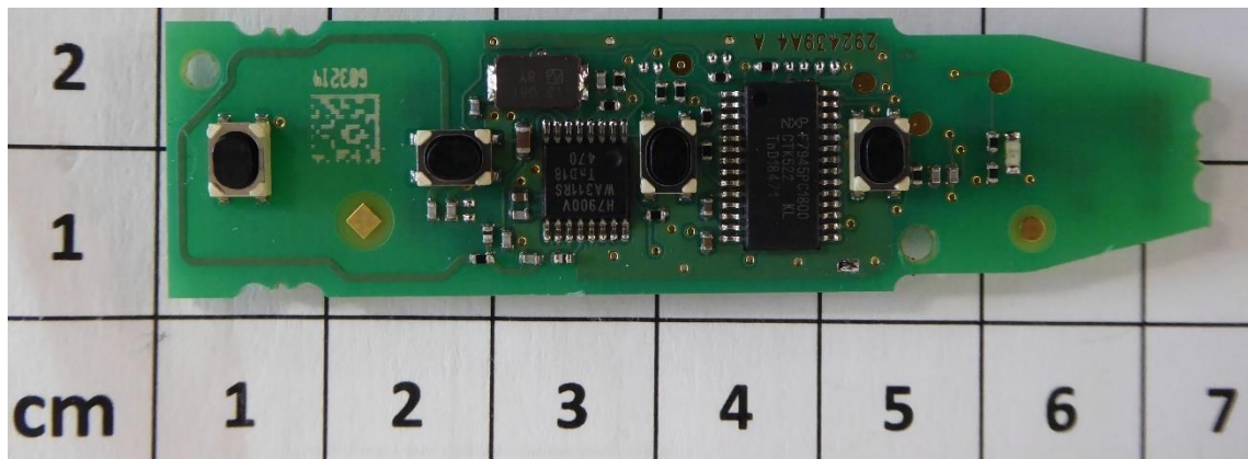
PCB bottom
