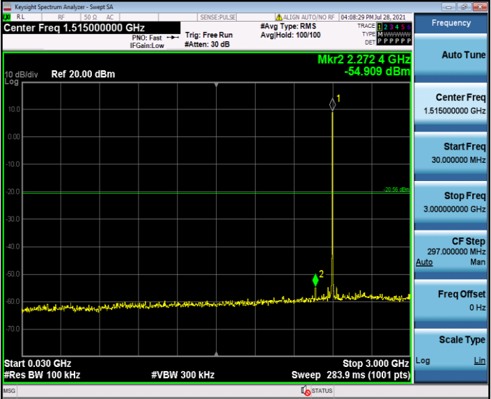
BLE_2402_30~3000
