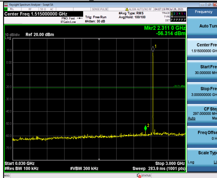
BLE 2440 30-3000
