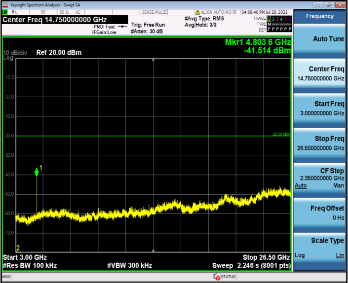
BLE_2402_3000~26500
