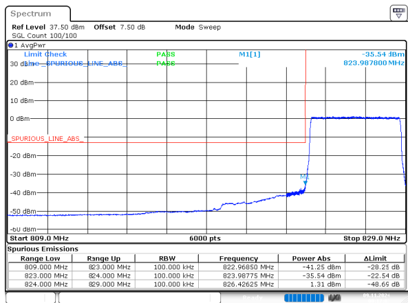
2_5MHz_Low_QPSK_25@0
