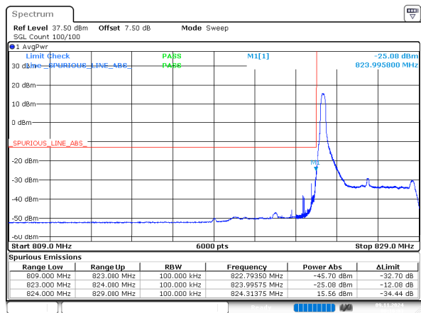
2_5MHz_Low_QPSK_1@0
