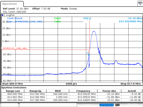
1_3MHz_Low_QPSK_1@0
