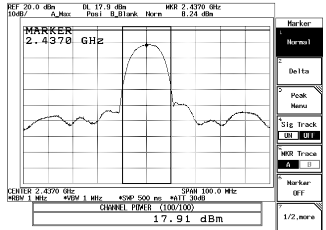
11Mbps-Ch06
