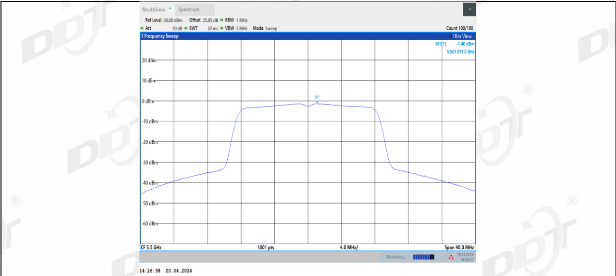
11A-CDD_Ant2_5500
