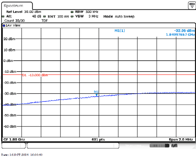
Band2-20MHz-16QAM-18700-1RB#24
