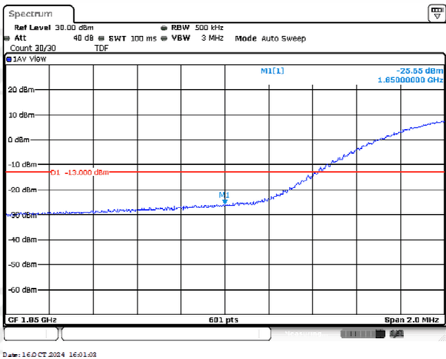
Band2-20MHz-16QAM-18700-25RB#0
