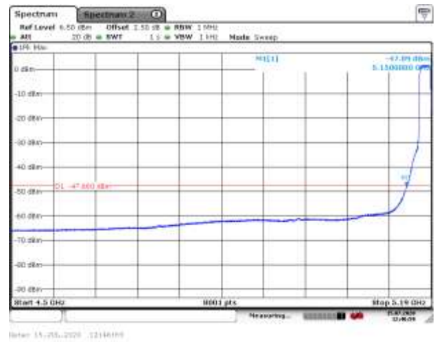
5200MHz AV
