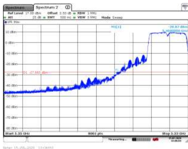
5550MHz PK
