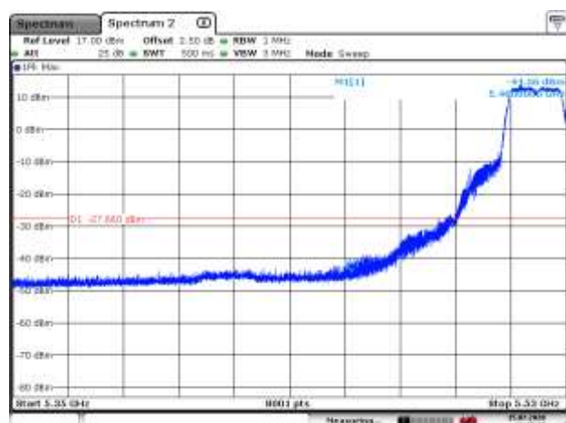
5520MHz PK
