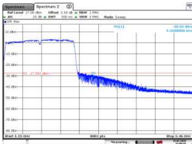
5290MHz PK
