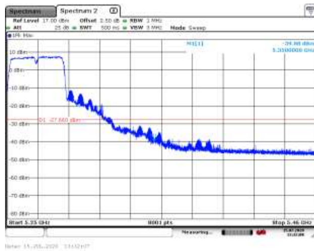
5270MHz PK
