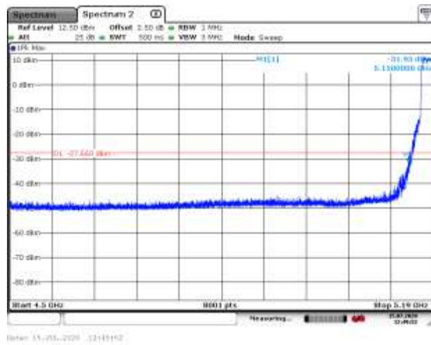
5200MHz PK
