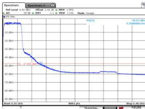
5320MHz AV
