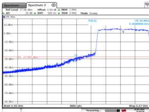
5530MHz PK
