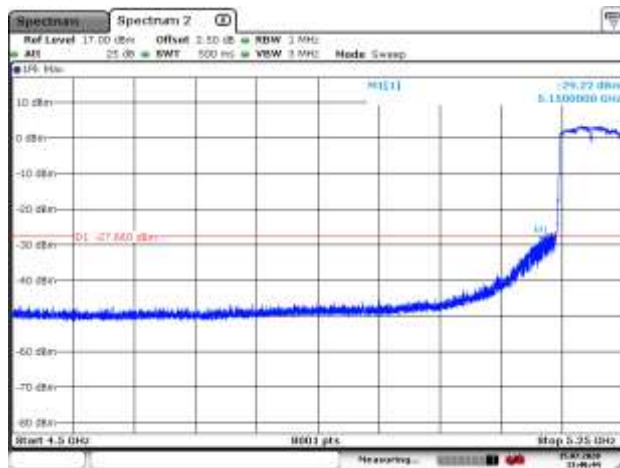
5210MHz PK
