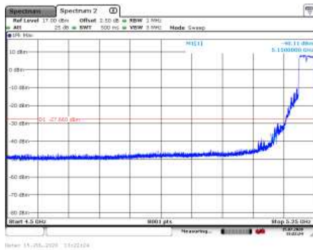
5270MHz PK
