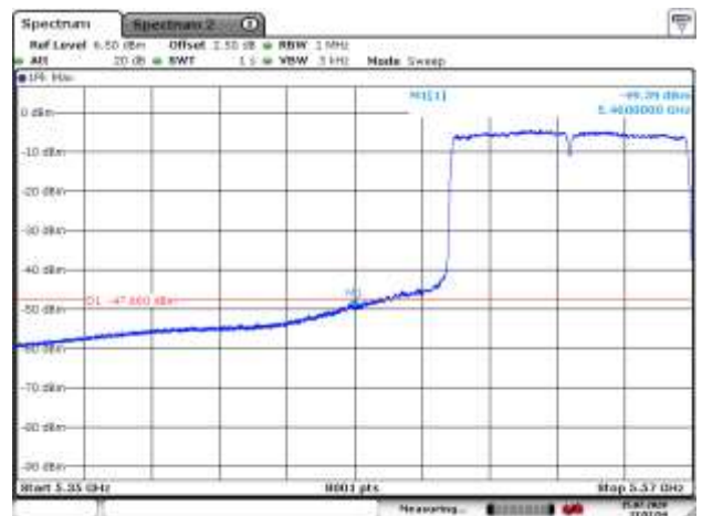
5530MHz AV
