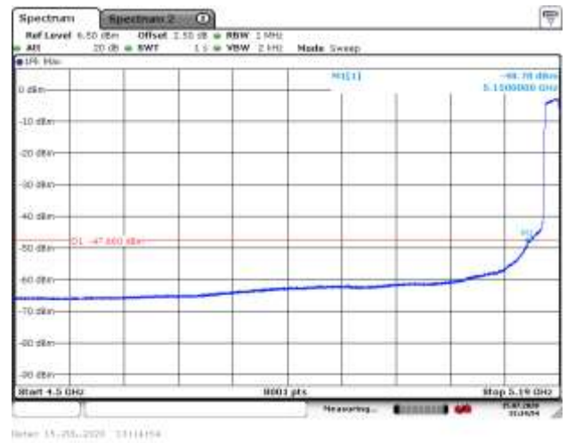
5230MHz AV
