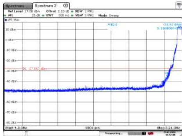
5200MHz PK
