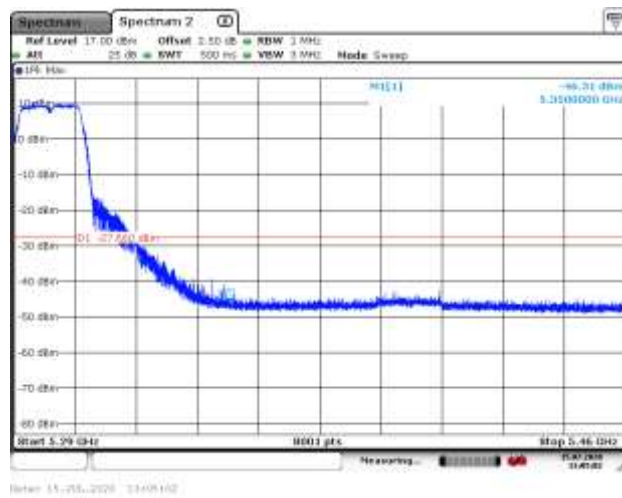
5300MHz PK
