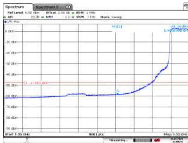
5520MHz AV
