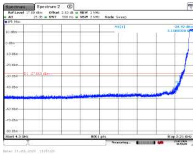
5300MHz PK
