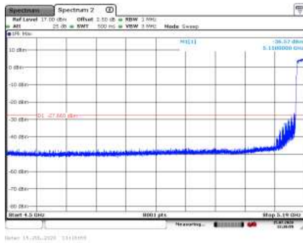
5230MHz PK
