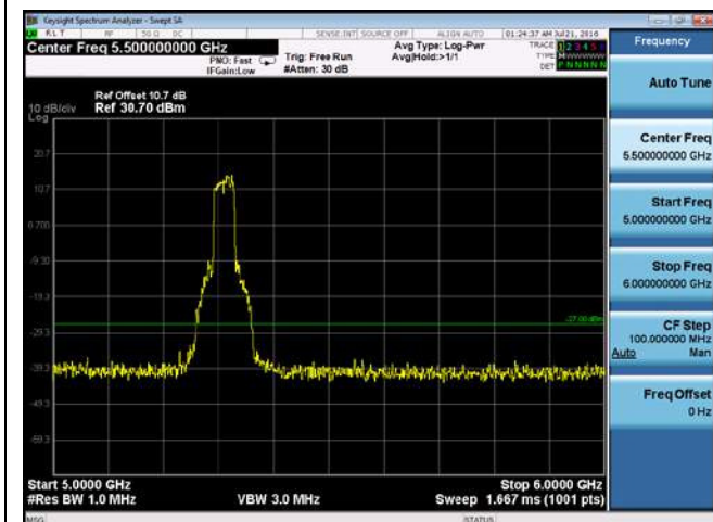
CUE-802.11n-40-5270M-chain3(5GHz-6GHz)
