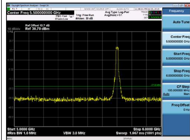
CUE-802.11n-20-5700M-chain 1(5GHz-6GHz)
