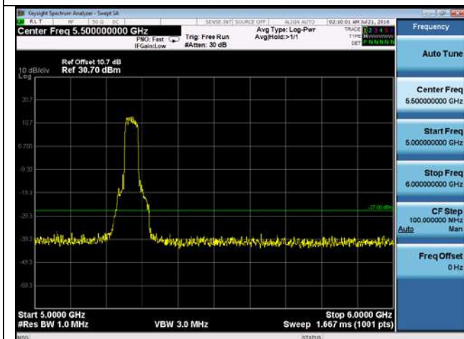
CUE-802.11n-40-5270M-chain4(5GHz-6GHz)
