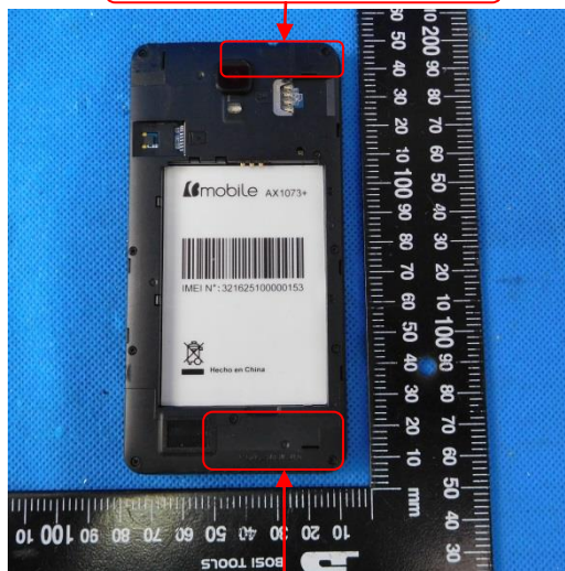
BT/WIFI ANT
