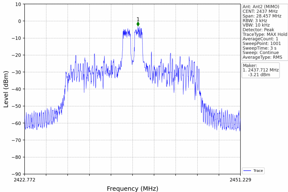
802.11ax(HEW20)_MCH_2437MHz_RU26_Mid_MIMO_NTNV
