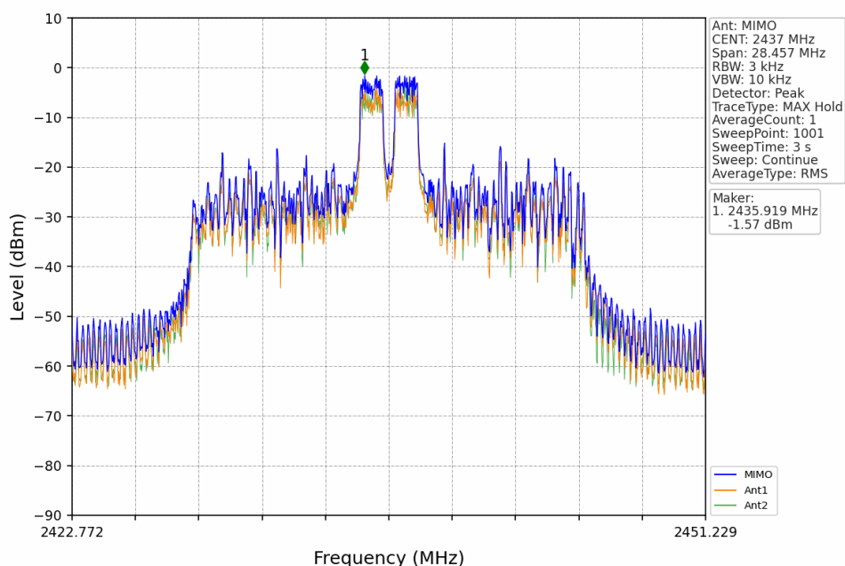
802.11ax(HEW20)_MCH_2437MHz_RU26_Mid_MIMO_NTNV
