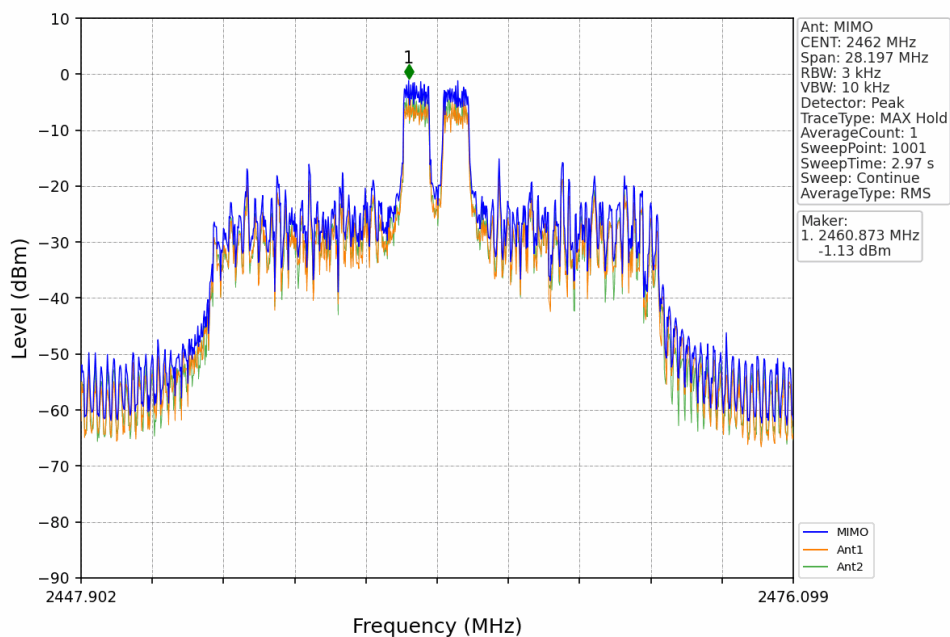
802.11ax(HEW20)_HCH_2462MHz_RU26_Mid_MIMO_NTNV
