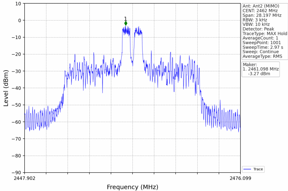
802.11ax(HEW20)_HCH_2462MHz_RU26_Mid_MIMO_NTNV
