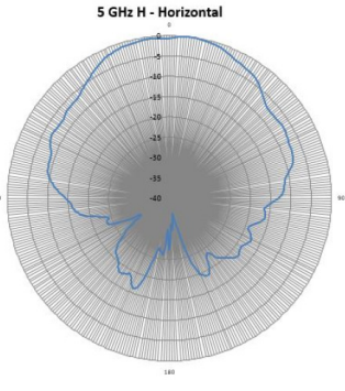
H-Plane Pattern
