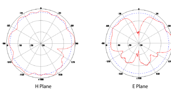
Port 2: 5500MHz
