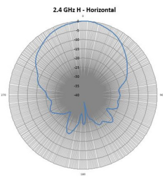
H-Plane Pattern
