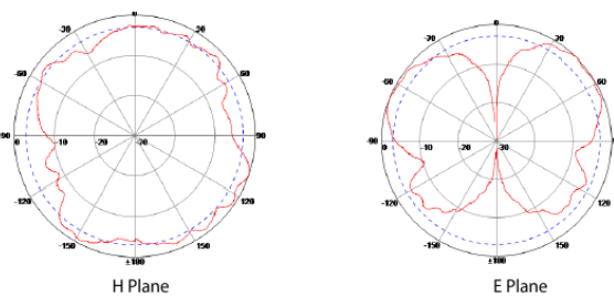
Port 3: 5500MHz
