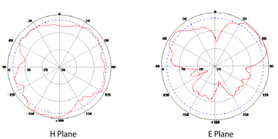
Port 2: 5500MHz
