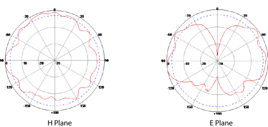
Port 4: 5500MHz
