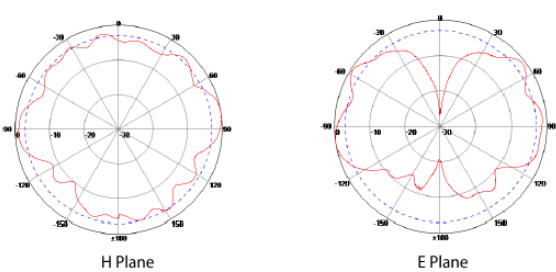
Port 1: 5500MHz
