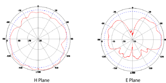
Port 3: 2450MHz
