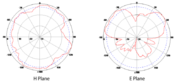
Port 2: 5500MHz
