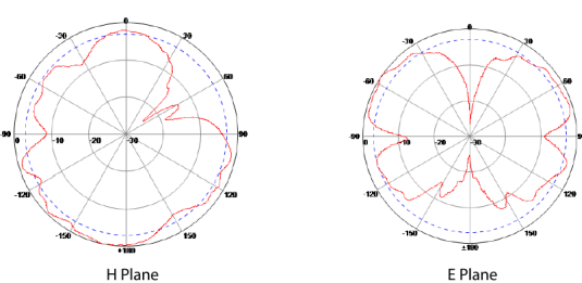
Port 4: 5500MHz
