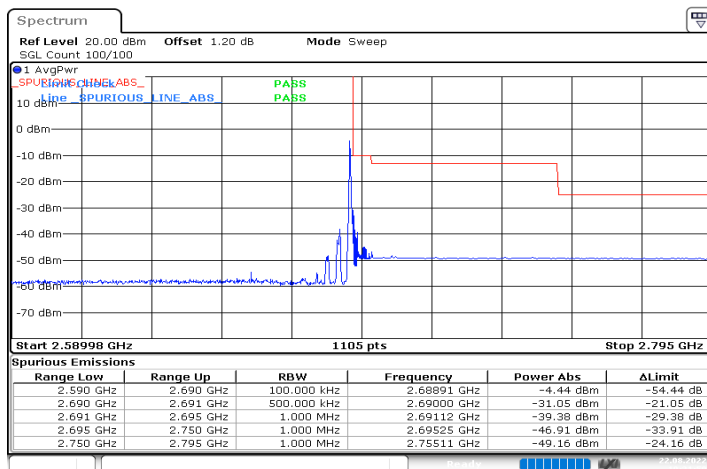
n41_60MHz_30kHz_2659.98MHz_DFT-s-OFDM QPSK_RB1@161
