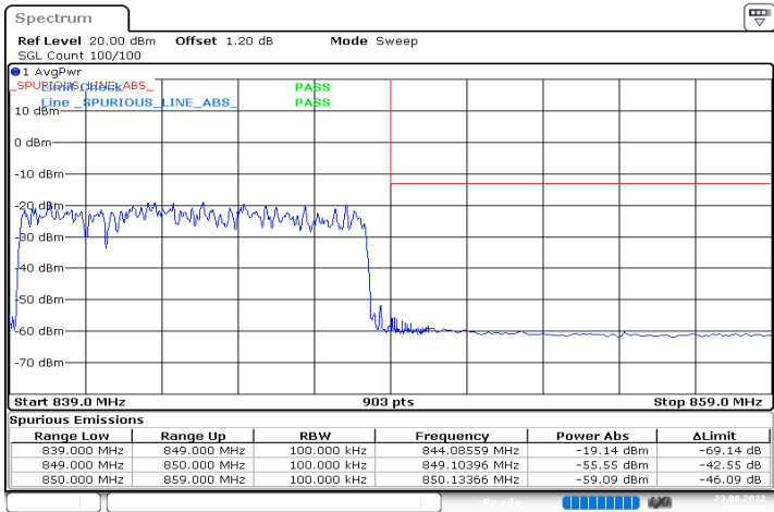
n5_10MHz_15kHz_844MHz_DFT-s-OFDM QPSK_RB50@0
