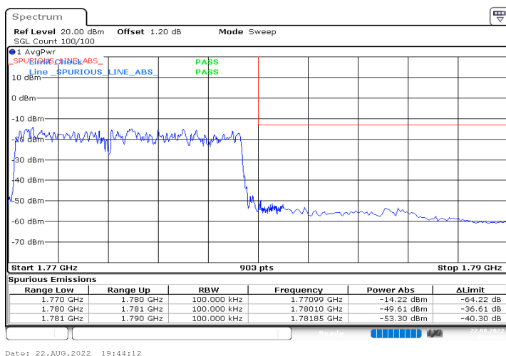
n66_10MHz_15kHz_1775MHz_DFT-s-OFDM QPSK_RB50@0
