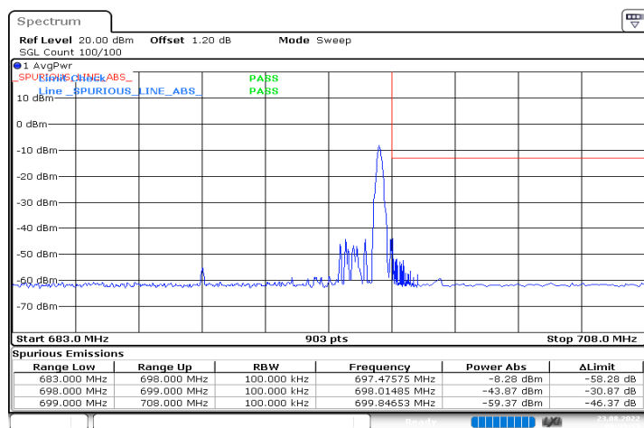
n71_15MHz_15kHz_690.5MHz_DFT-s-OFDM QPSK_RB1@78
