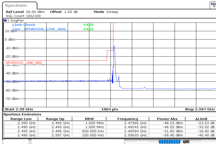
n41_60MHz_30kHz_2526MHz_DFT-s-OFDM QPSK_RB1@0
