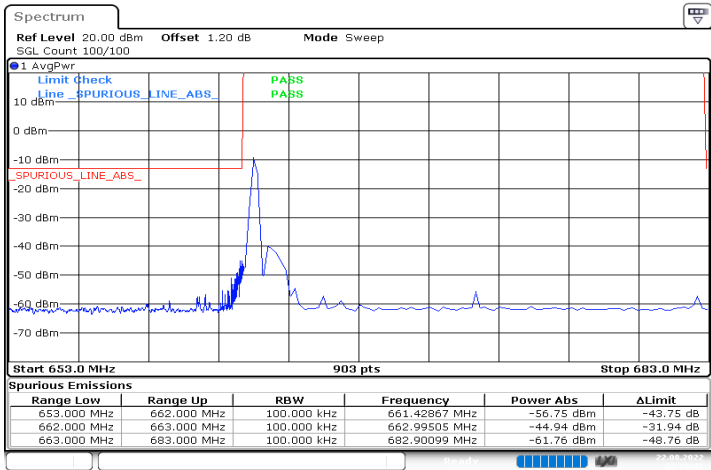
n71_20MHz_15kHz_673MHz_DFT-s-OFDM QPSK_RB1@0
