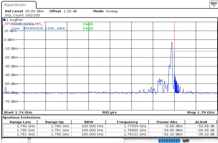
n66_40MHz_15kHz_1760MHz_DFT-s-OFDM QPSK_RB1@215
