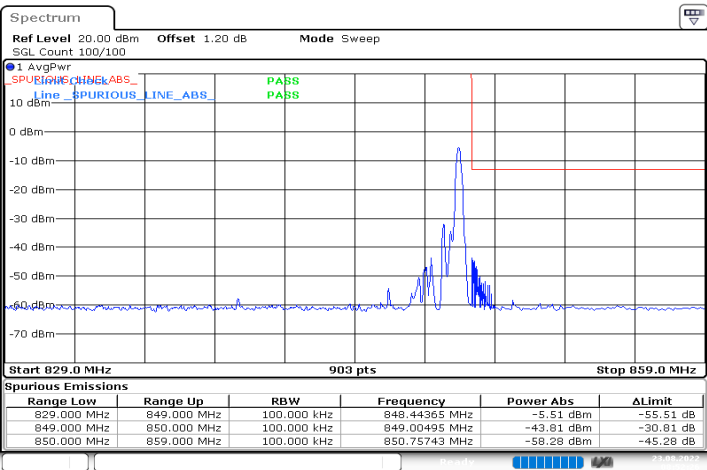
n5_20MHz_15kHz_839MHz_DFT-s-OFDM QPSK_RB1@105
