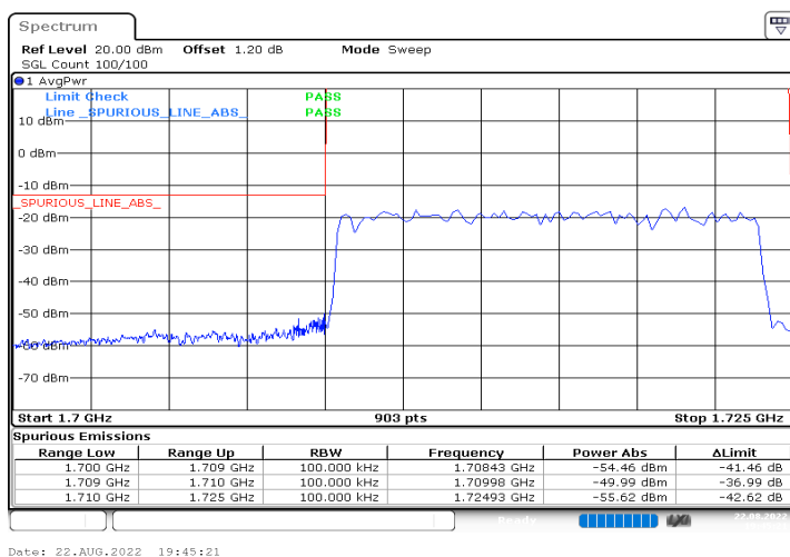
n66_15MHz_15kHz_1717.5MHz_DFT-s-OFDM QPSK_RB75@0
