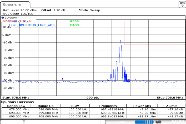
n71_20MHz_15kHz_688MHz_DFT-s-OFDM QPSK_RB1@105
