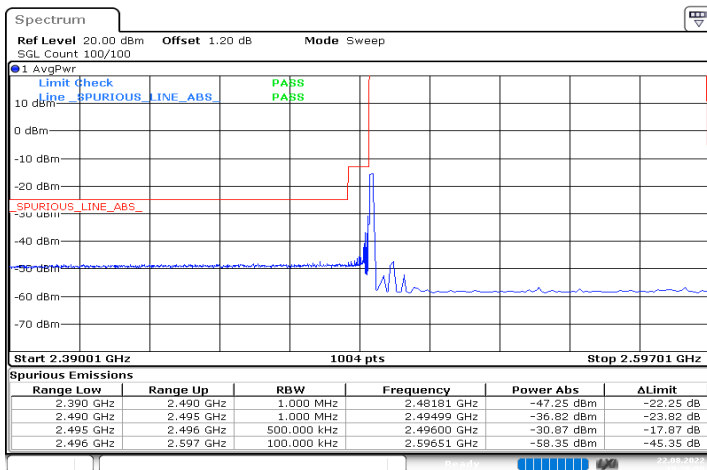
n41_100MHz_30kHz_2546.01MHz_DFT-s-OFDM QPSK_RB1@0
