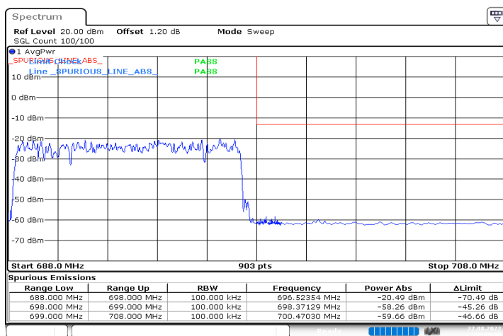
n71_10MHz_15kHz_693MHz_DFT-s-OFDM QPSK_RB50@0
