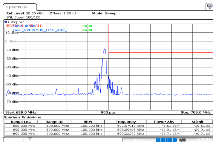
n71_10MHz_15kHz_693MHz_DFT-s-OFDM QPSK_RB1@51
