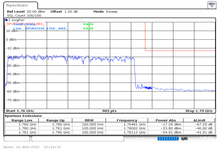
n66_20MHz_15kHz_1770MHz_DFT-s-OFDM QPSK_RB100@0
