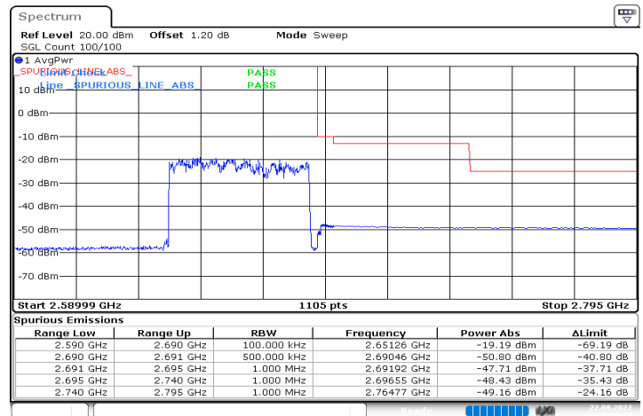
n41_50MHz_30kHz_2664.99MHz_DFT-s-OFDM QPSK_RB128@0
