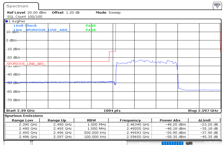
n41_60MHz_30kHz_2526MHz_DFT-s-OFDM QPSK_RB162@0
