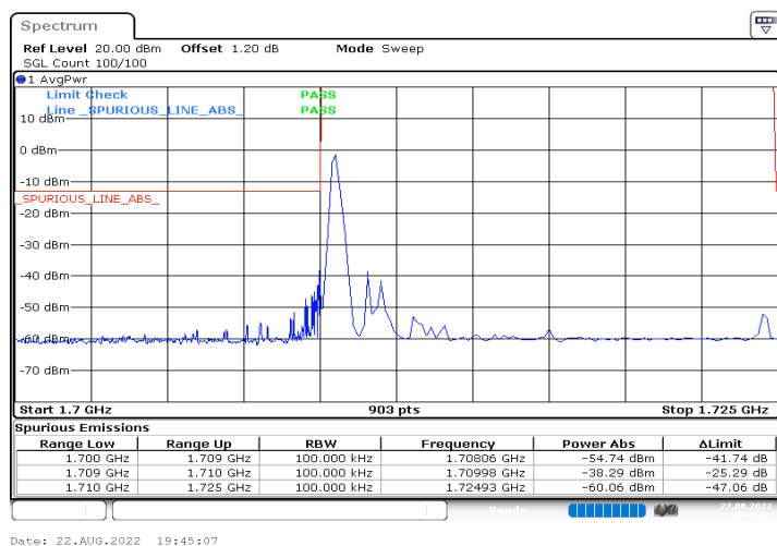
n66_15MHz_15kHz_1717.5MHz_DFT-s-OFDM QPSK_RB1@0
