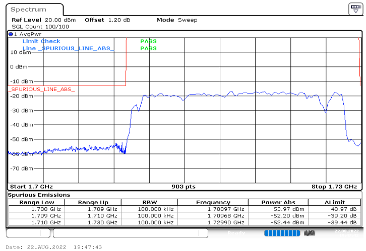
n66_20MHz_15kHz_1720MHz_DFT-s-OFDM QPSK_RB100@0
