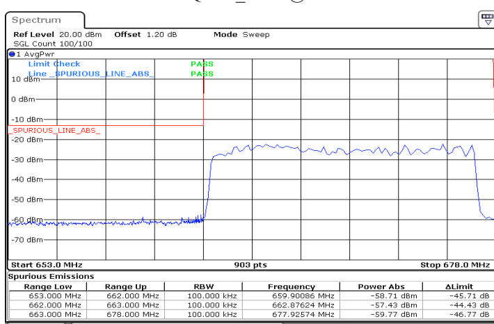
n71_15MHz_15kHz_670.5MHz_DFT-s-OFDM QPSK_RB75@0
