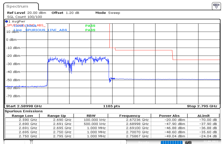
n41_60MHz_30kHz_2659.98MHz_DFT-s-OFDM QPSK_RB162@0
