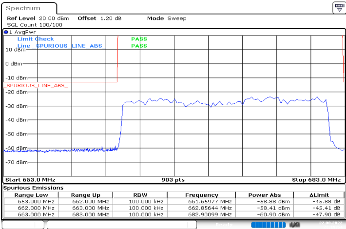
n71_20MHz_15kHz_673MHz_DFT-s-OFDM QPSK_RB100@0
