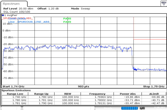
n66_40MHz_15kHz_1760MHz_DFT-s-OFDM QPSK_RB216@0
