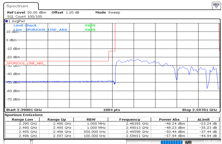
n41_100MHz_30kHz_2546.01MHz_DFT-s-OFDM QPSK_RB270@0
