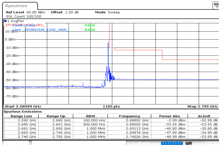
n41_50MHz_30kHz_2664.99MHz_DFT-s-OFDM QPSK_RB1@132
