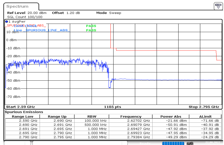
n41_100MHz_30kHz_2640MHz_DFT-s-OFDM QPSK_RB270@0
