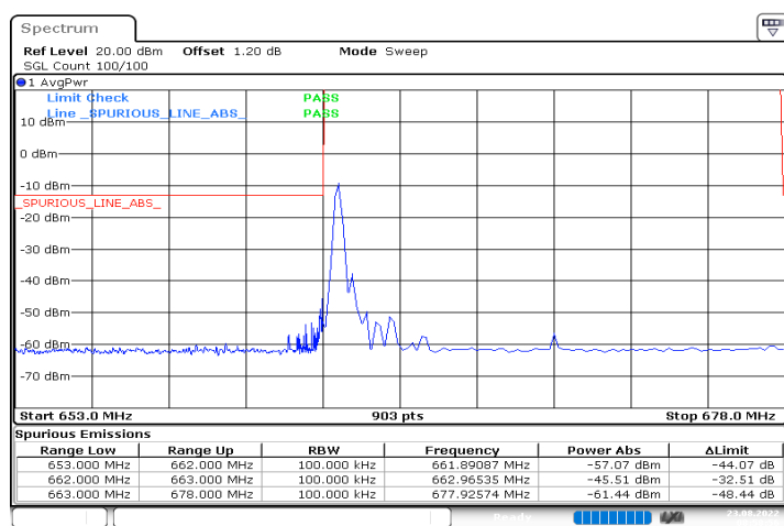
n71_15MHz_15kHz_670.5MHz_DFT-s-OFDM QPSK_RB1@0
