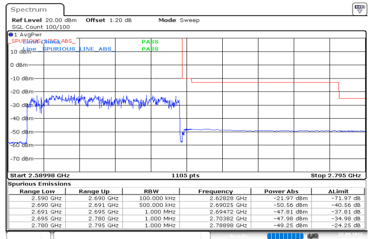
n41_90MHz_30kHz_2644.98MHz_DFT-s-OFDM QPSK_RB243@0
