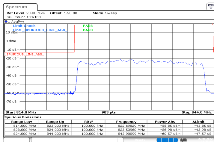
n5_20MHz_15kHz_834MHz_DFT-s-OFDM QPSK_RB100@0
