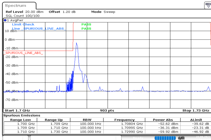
n66_20MHz_15kHz_1720MHz_DFT-s-OFDM QPSK_RB1@0
