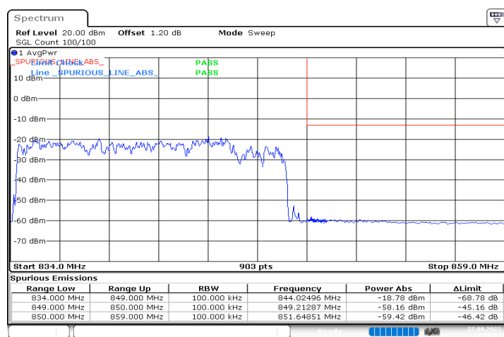
n5_15MHz_15kHz_841.5MHz_DFT-s-OFDM QPSK_RB75@0
