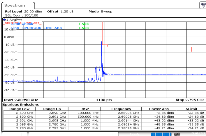
n41_90MHz_30kHz_2644.98MHz_DFT-s-OFDM QPSK_RB1@244
