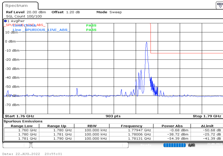
n66_20MHz_15kHz_1770MHz_DFT-s-OFDM QPSK_RB1@105
