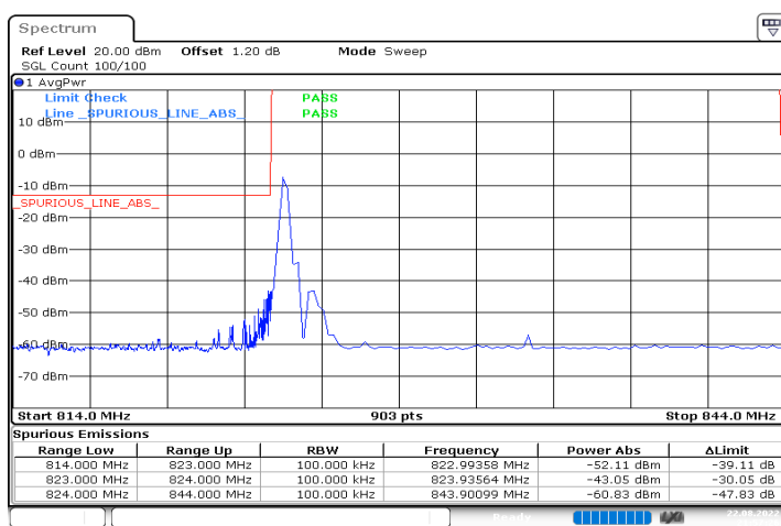
n5_20MHz_15kHz_834MHz_DFT-s-OFDM QPSK_RB1@0
