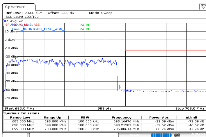
n71_15MHz_15kHz_690.5MHz_DFT-s-OFDM QPSK_RB75@0
