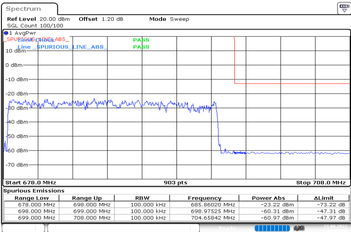
n71_20MHz_15kHz_688MHz_DFT-s-OFDM QPSK_RB100@0
