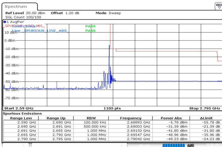
n41_100MHz_30kHz_2640MHz_DFT-s-OFDM QPSK_RB1@272
