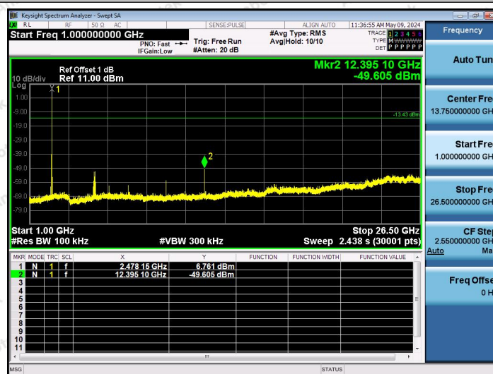
2.4G-Ant1-2479-1000~26500-PASS
