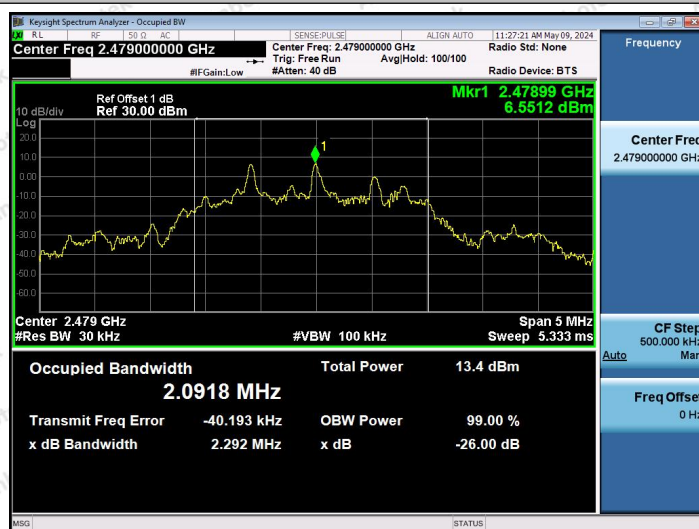
2.4G-Ant1-2479
