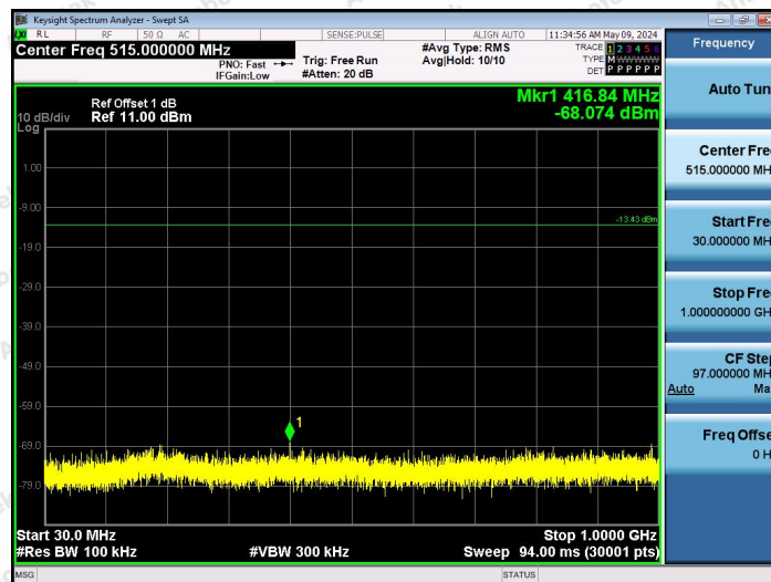
2.4G-Ant1-2479-30~1000-PASS
