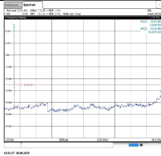
Band38-20MHz-QPSK-38000-1RB#0- Range2:1000~26500MHz
