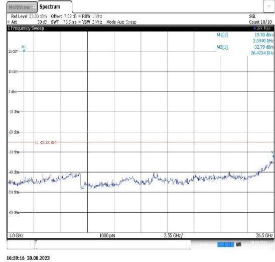
Band41-5MHz-QPSK-41565-1RB#0- Range2:1000~26500MHz
