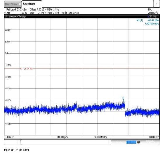
Band26(824-849)-15MHz-QPSK-26965-1RB#0-Range2:1000~10000MHz
