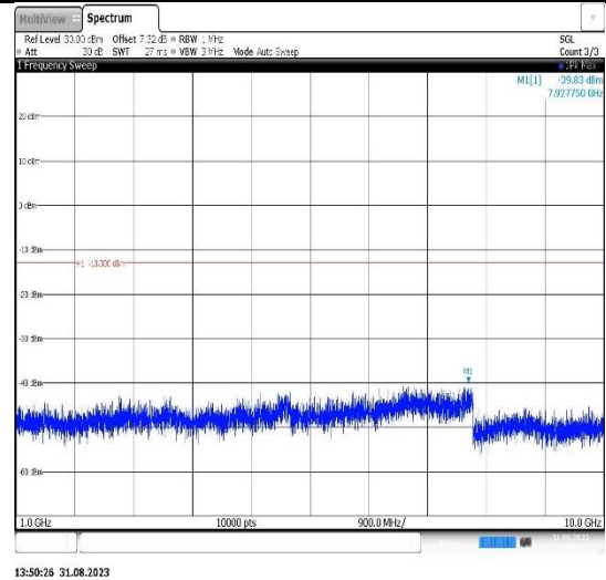
Band26(824-849)-15MHz-QPSK-26915-1RB#0-Range2:1000~10000MHz
