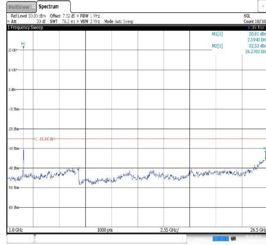
Band41-20MHz-QPSK-40620-1RB#0- Range2:1000~26500MHz
