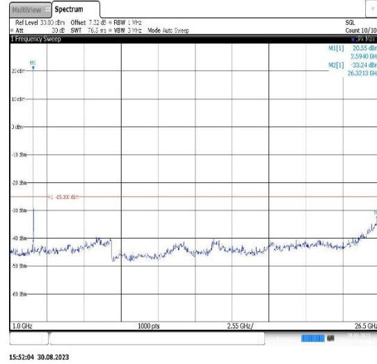
Band38-20MHz-QPSK-38150-1RB#0- Range2:1000~26500MHz
