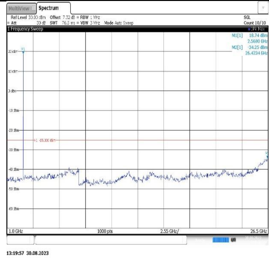
Band38-5MHz-QPSK-38000-1RB#0- Range2:1000~26500MHz
