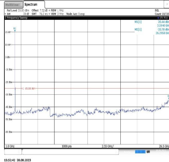
Band38-20MHz-16QAM-37850-1RB#0- Range2:1000~26500MHz
