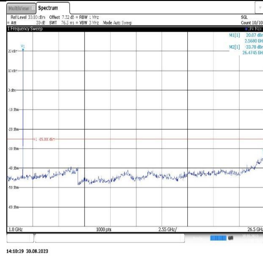
Band38-10MHz-QPSK-38000-1RB#0- Range2:1000~26500MHz
