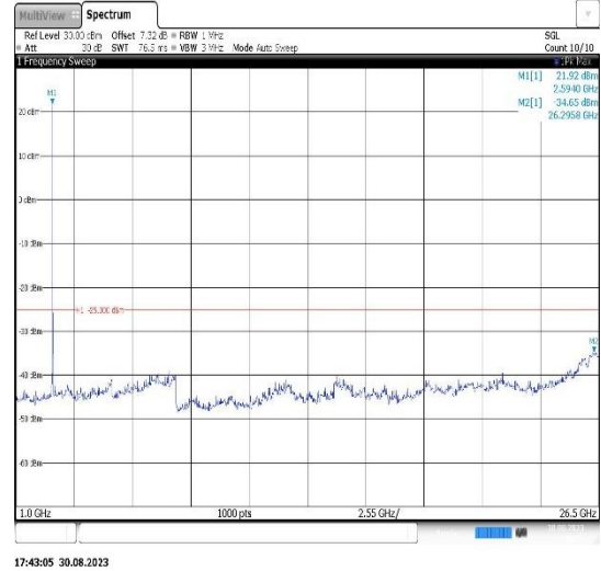
Band41-10MHz-QPSK-41540-1RB#0- Range2:1000~26500MHz
