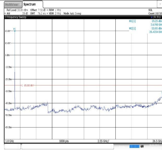
Band41-20MHz-QPSK-41490-1RB#0- Range2:1000~26500MHz
