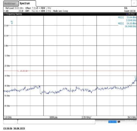
Band38-5MHz-QPSK-38225-1RB#0- Range2:1000~26500MHz
