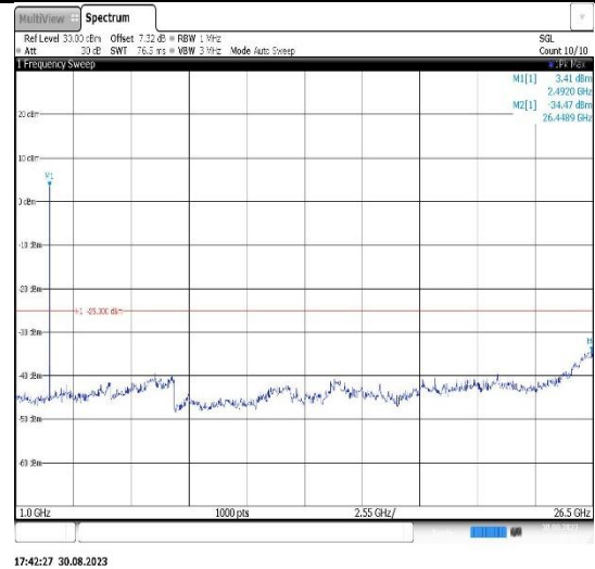
Band41-10MHz-QPSK-40620-1RB#0- Range2:1000~26500MHz
