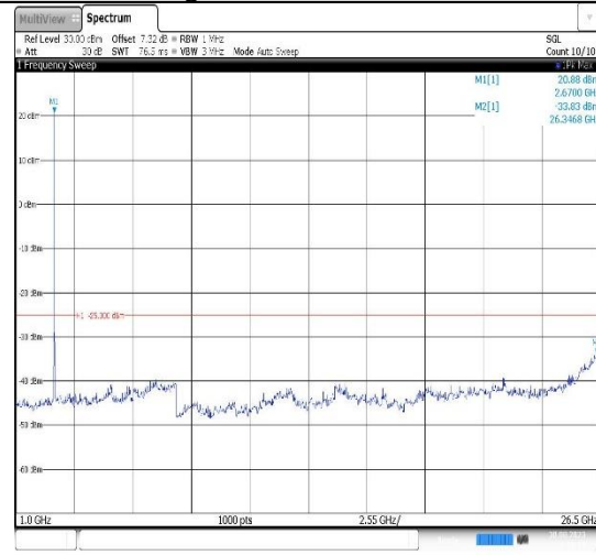
Band41-15MHz-QPSK-41515-1RB#0- Range2:1000~26500MHz
