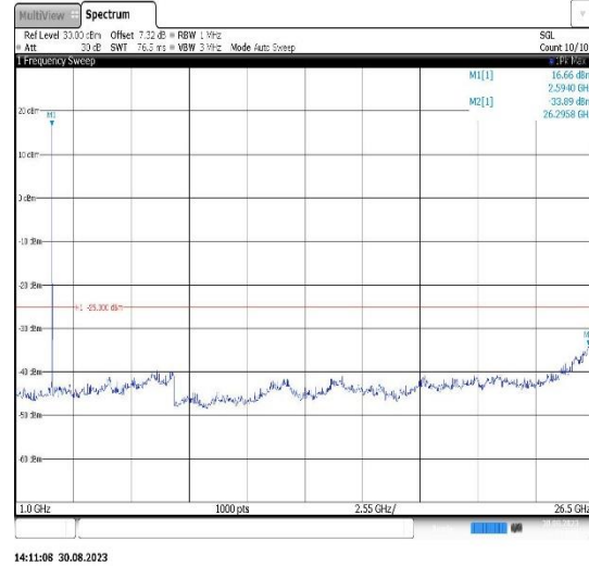
Band38-10MHz-QPSK-38200-1RB#0- Range2:1000~26500MHz
