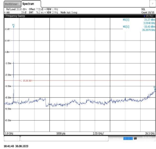
Band41-20MHz-16QAM-41490-1RB#0- Range2:1000~26500MHz
