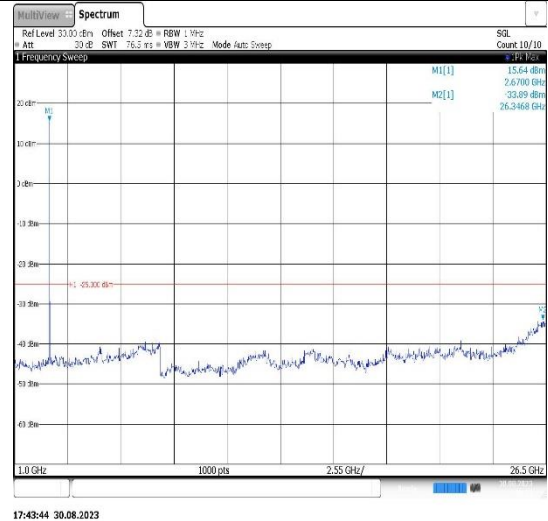
Band41-10MHz-16QAM-39700-1RB#0- Range2:1000~26500MHz
