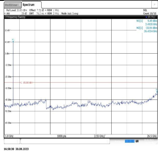
Band41-5MHz-QPSK-40620-1RB#0- Range2:1000~26500MHz
