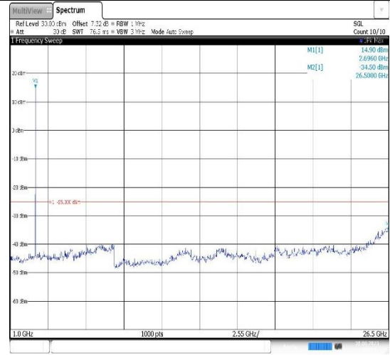
Band41-5MHz-16QAM-41565-1RB#0- Range2:1000~26500MHz
