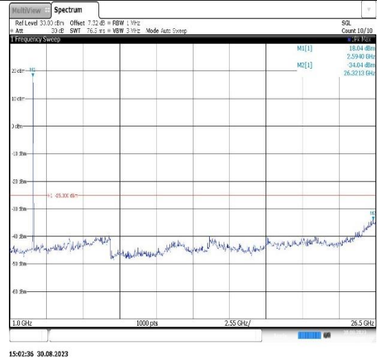
Band38-20MHz-QPSK-37850-1RB#0- Range2:1000~26500MHz
