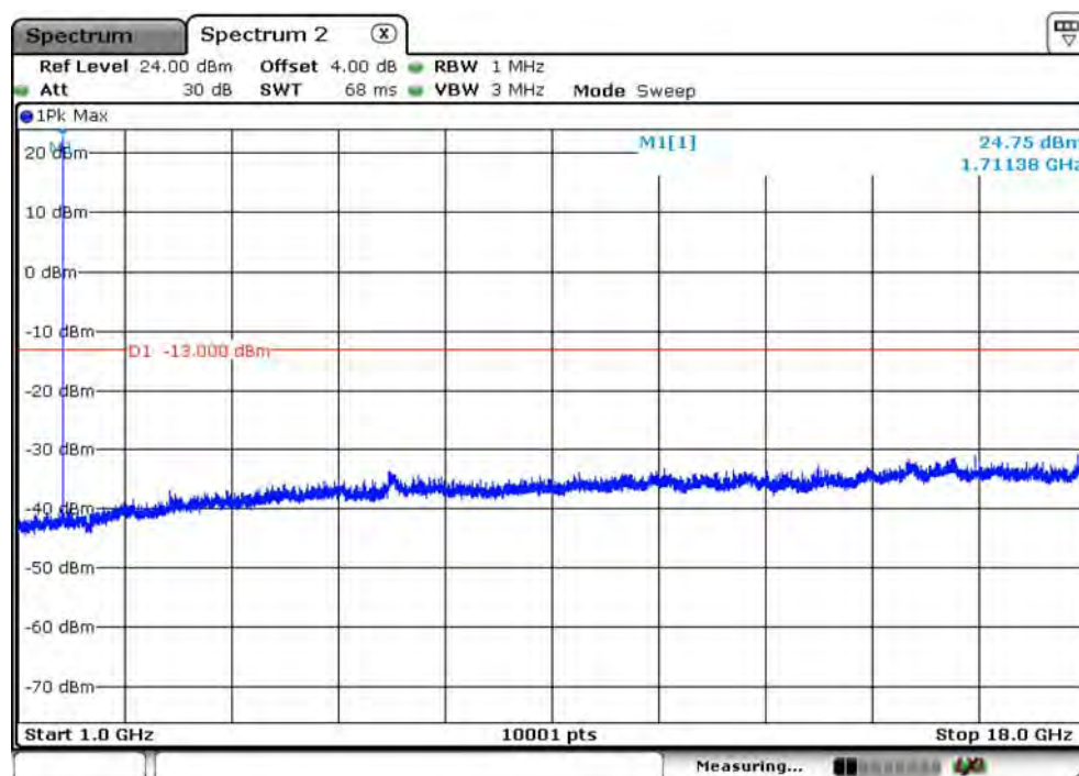
B66_CH131979_1.4M_1RB2_QPSK_Above 1G
