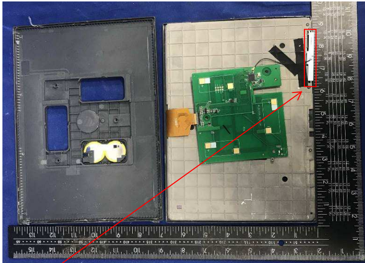
Antenna
