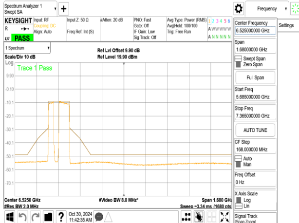
802.11be_160MHz_ChainA_6025MHz_996+484_MRUI4
