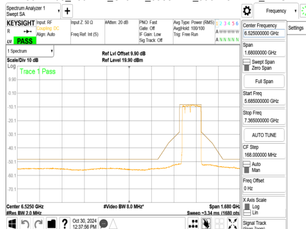
802.11be_160MHz_ChainB_6985MHz_996+484+242_MRU2
