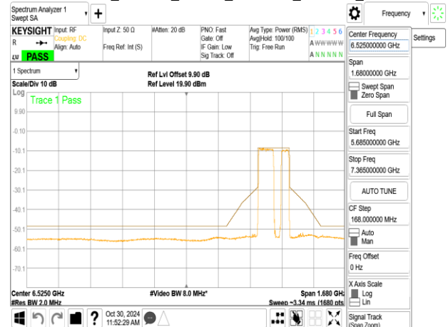
802.11be_160MHz_ChainA_6985MHz_996+484_MRU3
