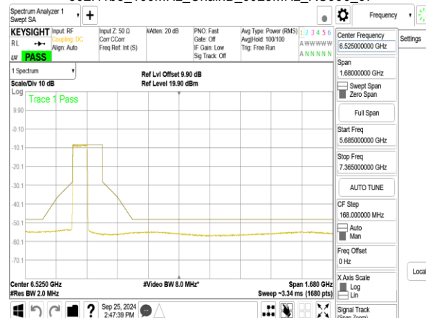
802.11be_160MHz_ChainB_6185MHz
