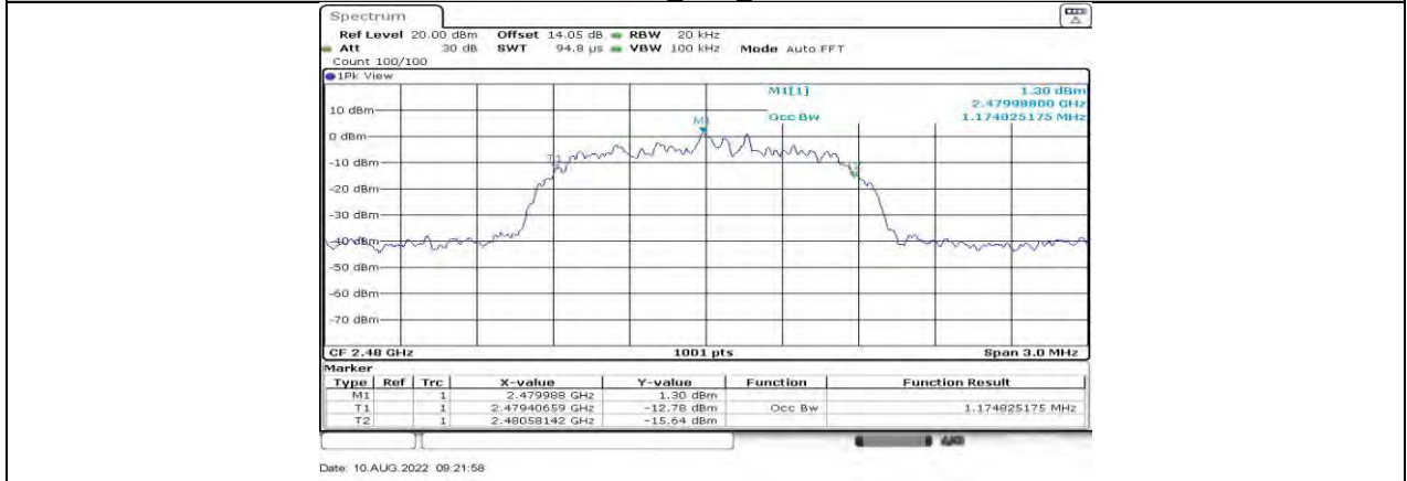
2DH5_Ant1_2480
