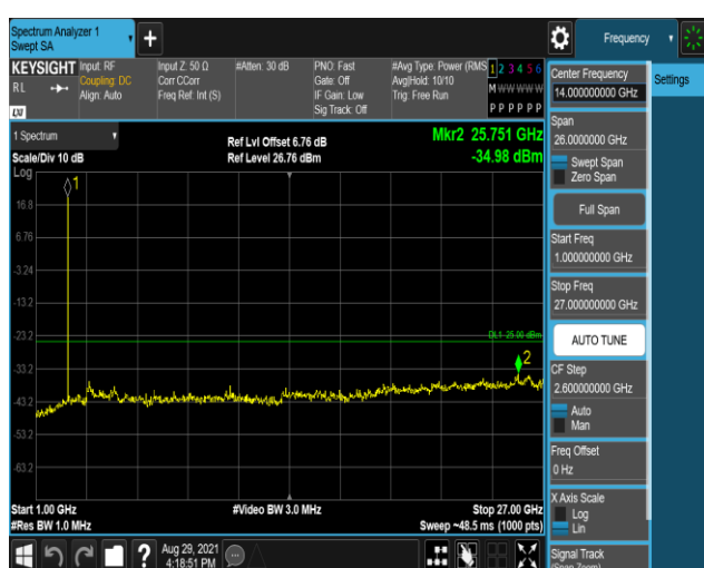
Band41-20MHz-QPSK-41140:1000~27000MHz
