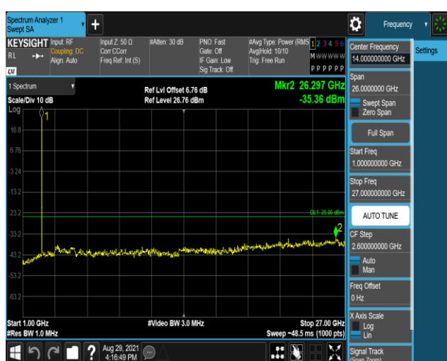
Band41-20MHz-OPSK-40640:1000~27000MHz
