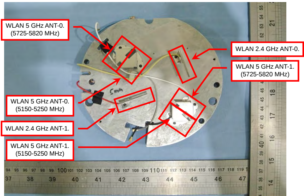
EUT Photo (4)
