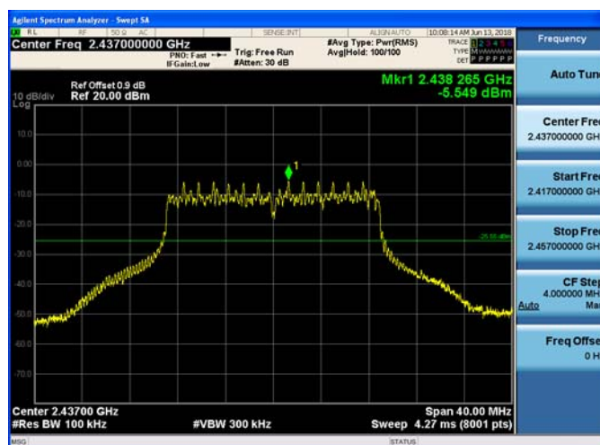
802.11n(HT20) CH06
