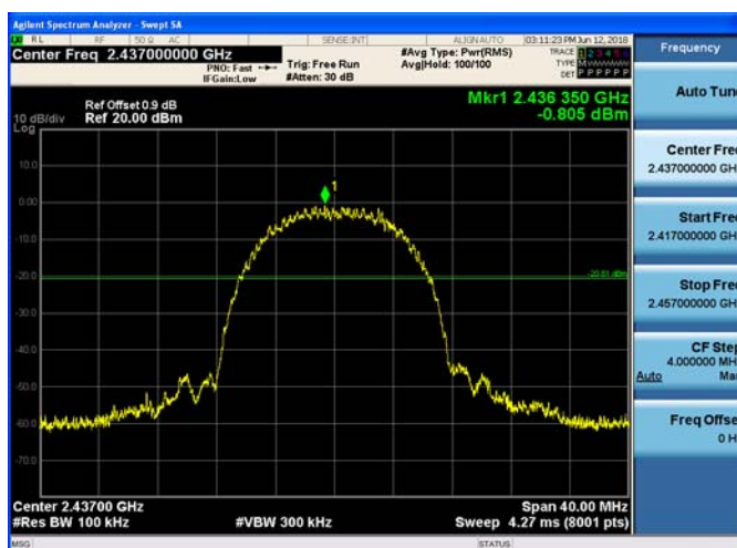
802.11b CH06
