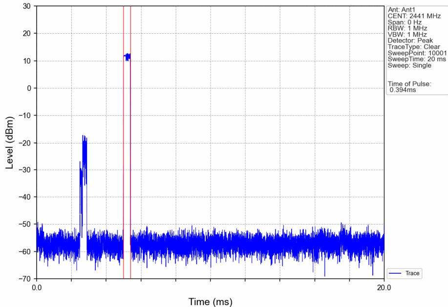
8DPSK_3DH1_HOPP_Ant1_NTNV
