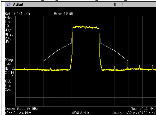
6665MHz_143_160MHz BW_be-mode_Chain 0
