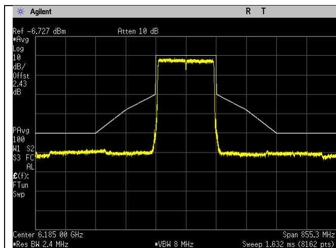
6185MHz_47_160MHz BW_be-mode_Chain 2
