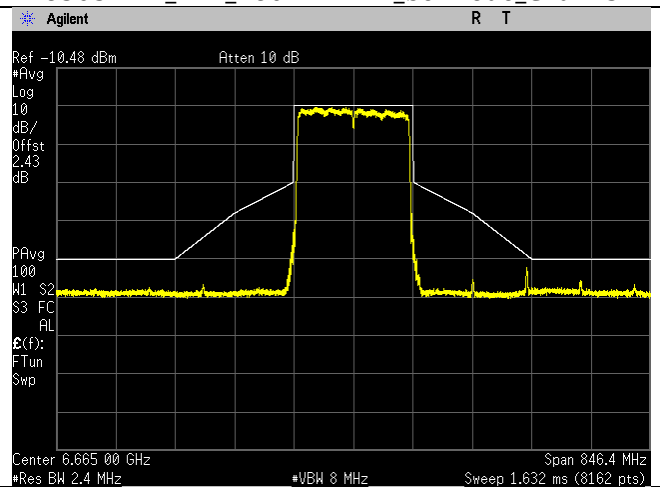
6665MHz_143_160MHz BW_be-mode_Chain 1
