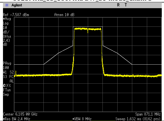
6185MHz_47_160MHz BW_be-mode_Chain 1
