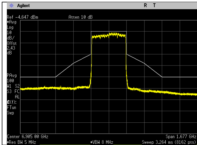
6905MHz_191_320MHz BW_be-mode_Chain 0
