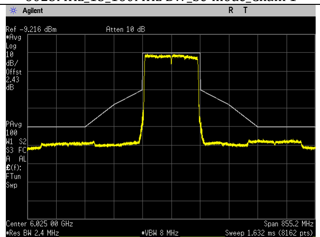
6025MHz_15_160MHz BW_be-mode_Chain 3
