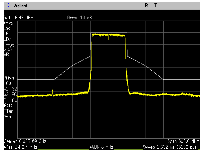
6025MHz_15_160MHz BW_be-mode_Chain 1
