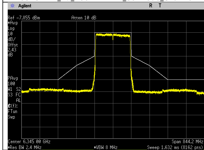
6345MHz_79_160MHz BW_be-mode_Chain 2
